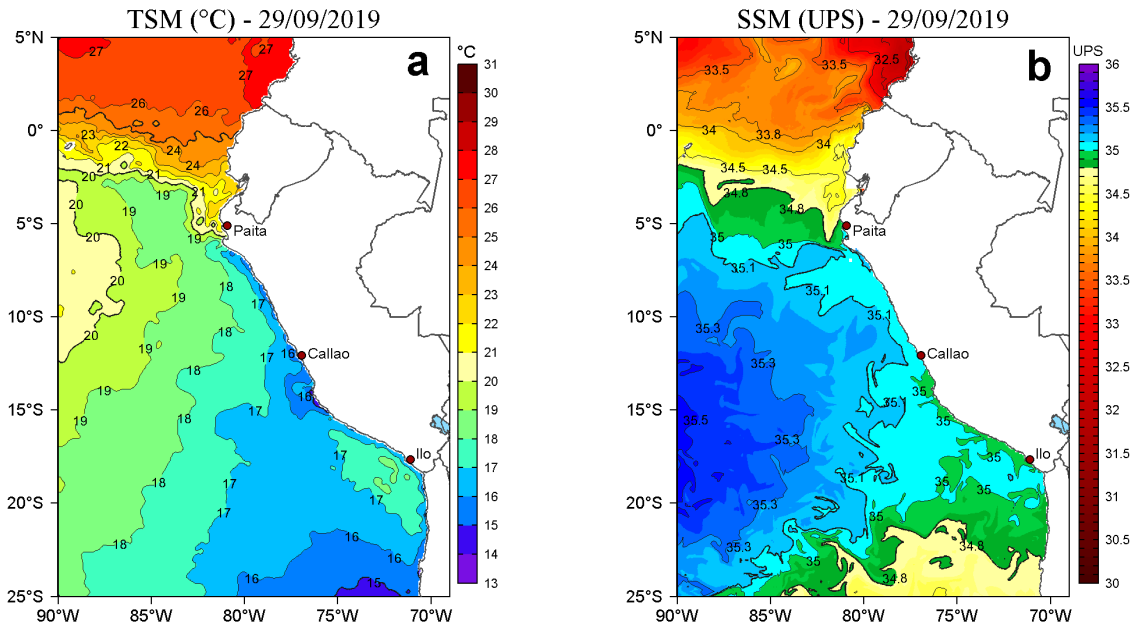
Figura 2. a) Temperatura superficial del mar (TSM, °C) y b) Salinidad superficial del mar (SSM, UPS), para el 29 de setiembre de 2019. Datos: OSTIA-UKMO-L4-GLOB-v2.0 (UK Met Office, 2012; Donlon et al, 2012) disponible en https://podaac.jpl.nasa.gov/dataset/OSTIA-UKMO-L4-GLOB-v2.0 para (a) y Hybrid Coordinate Ocean Model v. GOFS 3.1 (HYCOM; Halliwell et al., 1998; 2000; Bleck, 2001) para (b). Procesamiento: LHF/AFIOF/DGIOCC/IMARPE.
