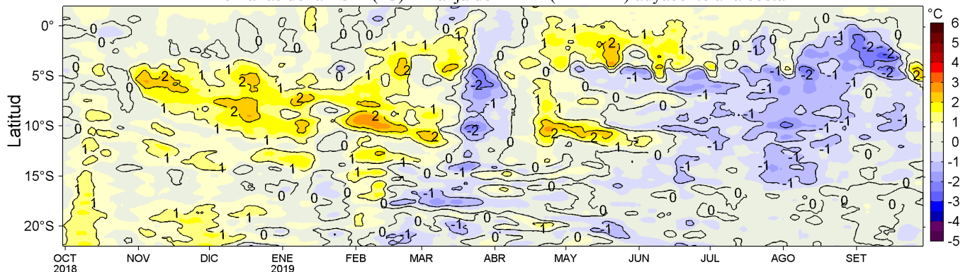
Figura 4. Variación promedio de las anomalías de la temperatura superficial del mar (TSM, °C) para una franja de 60 mn (~111 km) adyacente al litoral peruano para los últimos doce meses al 29 de setiembre de 2019. Datos: OSTIA-UKMO-L4-GLOB-v2.0 (UK Met. Office, 2012; Donlon et al, 2012) disponible en https://podaac.jpl.nasa.gov/dataset/OSTIA-UKMO-L4-GLOB-v2.0 . Las anomalías se calcularon con respecto al periodo 2007-2016. Procesamiento: LHF/AFIOF/DGIOCC/IMARPE.
