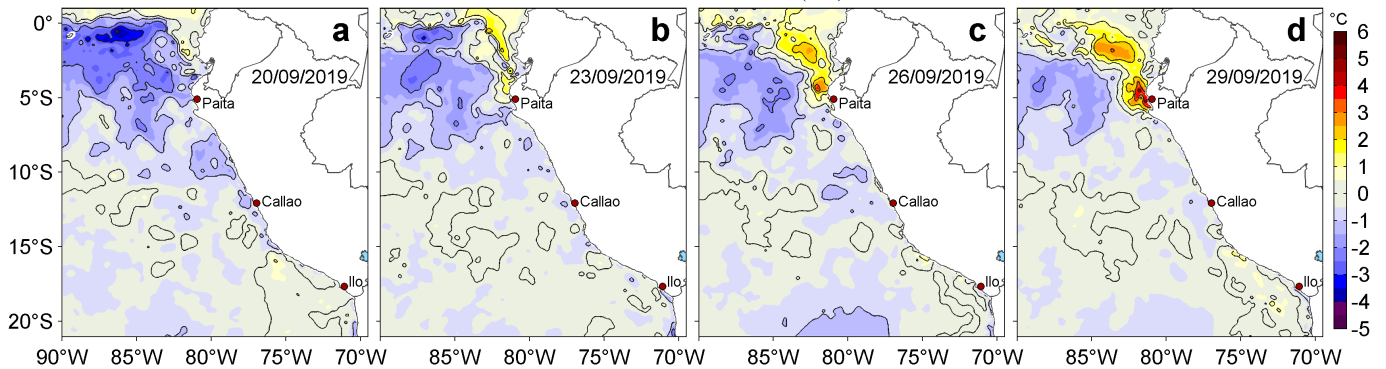
Figura 3. Anomalías de la temperatura superficial del mar (TSM, °C) para los días: a) 20, b) 23, c) 26 y d) 29 de setiembre de 2019. Las anomalías se calcularon respecto de la climatología para el periodo 2007-2016. Datos: OSTIA-UKMO-L4-GLOB-v2.0 (UK Met Office, 2012; Donlon et al, 2012). Procesamiento: LHF/AFIOF/DGIOCC/IMARPE.
