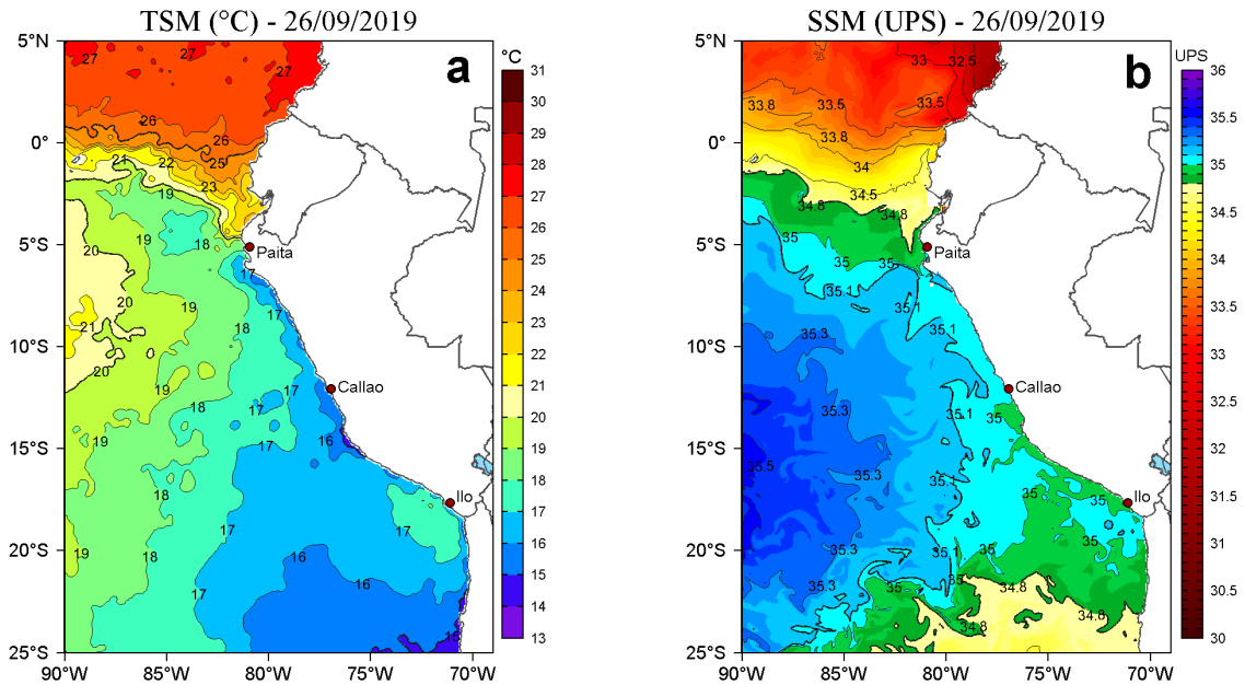
Figura 2. a) Temperatura superficial del mar (TSM, °C) y b) Salinidad superficial del mar (SSM, UPS), para el 26 de setiembre de 2019. Datos: OSTIA-UKMO-L4-GLOB-v2.0 (UK Met Office, 2012; Donlon et al, 2012) disponible en https://podaac.jpl.nasa.gov/dataset/OSTIA-UKMO-L4-GLOB-v2.0 para (a) y Hybrid Coordinate Ocean Model v. GOFS 3.1 (HYCOM; Halliwell et al., 1998; 2000; Bleck, 2001) para (b). Procesamiento: LHF/AFIOF/DGIOCC/IMARPE.
