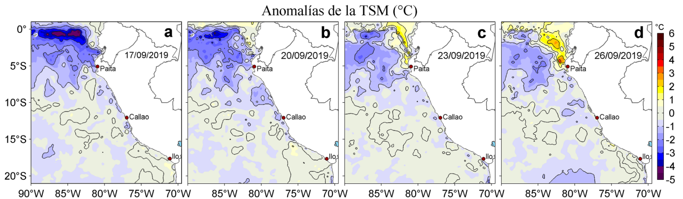
Figura 3. Anomalías de la temperatura superficial del mar (TSM, °C) para los días: a) 17, b) 20, c) 23 y d) 26 de setiembre de 2019. Las anomalías se calcularon respecto de la climatología para el periodo 2007-2016. Datos: OSTIA-UKMO-L4-GLOB-v2.0 (UK Met Office, 2012; Donlon et al, 2012). Procesamiento: LHF/AFIOF/DGIOCC/IMARPE.
