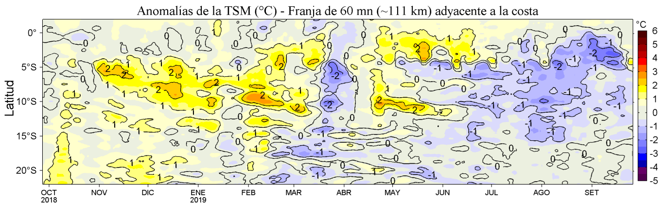
Figura 4. Variación promedio de las anomalías de la temperatura superficial del mar (TSM, °C) para una franja de 60 mn (~111 km) adyacente al litoral peruano para los últimos doce meses al 26 de setiembre de 2019. Datos: OSTIA-UKMO-L4-GLOB-v2.0 (UK Met. Office, 2012; Donlon et al, 2012) disponible en https://podaac.jpl.nasa.gov/dataset/OSTIA-UKMO-L4-GLOB-v2.0 . Las anomalías se calcularon con respecto al periodo 2007-2016. Procesamiento: LHF/AFIOF/DGIOCC/IMARPE.
