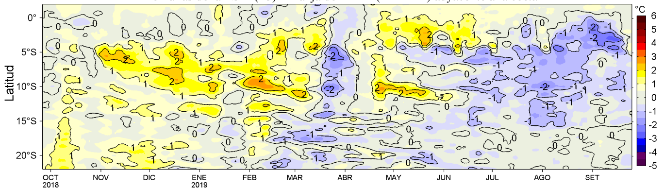
Figura 4. Variación promedio de las anomalías de la temperatura superficial del mar (TSM, °C) para una franja de 60 mn (~111 km) adyacente al litoral peruano para los últimos doce meses al 25 de setiembre de 2019. Datos: OSTIA-UKMO-L4-GLOB-v2.0 (UK Met. Office, 2012; Donlon et al, 2012) disponible en https://podaac.jpl.nasa.gov/dataset/OSTIA-UKMO-L4-GLOB-v2.0 . Las anomalías se calcularon con respecto al periodo 2007-2016. Procesamiento: LHF/AFIOF/DGIOCC/IMARPE.
