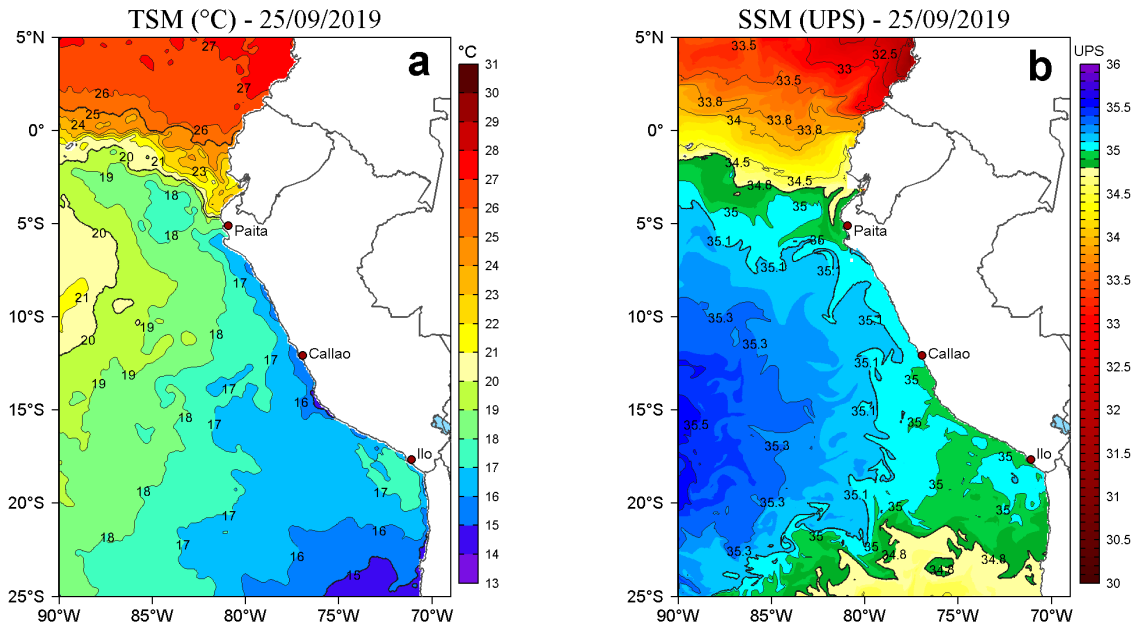
Figura 2. a) Temperatura superficial del mar (TSM, °C) y b) Salinidad superficial del mar (SSM, UPS), para el 25 de setiembre de 2019. Datos: OSTIA-UKMO-L4-GLOB-v2.0 (UK Met Office, 2012; Donlon et al, 2012) disponible en https://podaac.jpl.nasa.gov/dataset/OSTIA-UKMO-L4-GLOB-v2.0 para (a) y Hybrid Coordinate Ocean Model v. GOFS 3.1 (HYCOM; Halliwell et al., 1998; 2000; Bleck, 2001) para (b). Procesamiento: LHF/AFIOF/DGIOCC/IMARPE.
