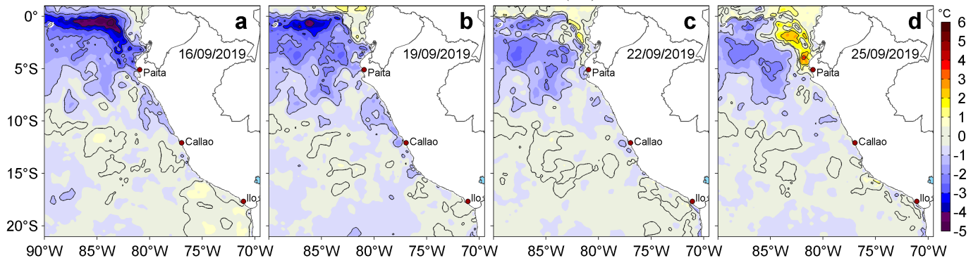
Figura 3. Anomalías de la temperatura superficial del mar (TSM, °C) para los días: a) 16, b) 19, c) 22 y d) 25 de setiembre de 2019. Las anomalías se calcularon respecto de la climatología para el periodo 2007-2016. Datos: OSTIA-UKMO-L4-GLOB-v2.0 (UK Met Office, 2012; Donlon et al, 2012). Procesamiento: LHF/AFIOF/DGIOCC/IMARPE.
