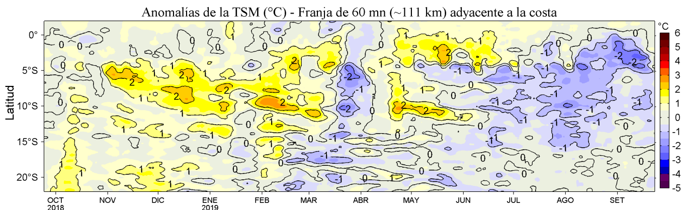
Figura 4. Variación promedio de las anomalías de la temperatura superficial del mar (TSM, °C) para una franja de 60 mn (~111 km) adyacente al litoral peruano para los últimos doce meses al 23 de setiembre de 2019. Datos: OSTIA-UKMO-L4-GLOB-v2.0 (UK Met. Office, 2012; Donlon et al, 2012) disponible en https://podaac.jpl.nasa.gov/dataset/OSTIA-UKMO-L4-GLOB-v2.0 . Las anomalías se calcularon con respecto al periodo 2007-2016. Procesamiento: LHF/AFIOF/DGIOCC/IMARPE.
