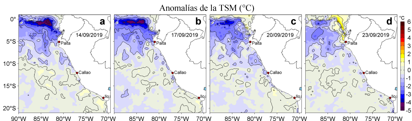
Figura 3. Anomalías de la temperatura superficial del mar (TSM, °C) para los días: a) 14, b) 17, c) 20 y d) 23 de setiembre de 2019. Las anomalías se calcularon respecto de la climatología para el periodo 2007-2016. Datos: OSTIA-UKMO-L4-GLOB-v2.0 (UK Met Office, 2012; Donlon et al, 2012). Procesamiento: LHF/AFIOF/DGIOCC/IMARPE.
