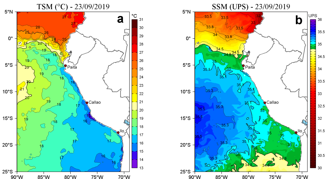
Figura 2. a) Temperatura superficial del mar (TSM, °C) y b) Salinidad superficial del mar (SSM, UPS), para el 23 de setiembre de 2019. Datos: OSTIA-UKMO-L4-GLOB-v2.0 (UK Met Office, 2012; Donlon et al, 2012) disponible en https://podaac.jpl.nasa.gov/dataset/OSTIA-UKMO-L4-GLOB-v2.0 para (a) y Hybrid Coordinate Ocean Model v. GOFS 3.1 (HYCOM; Halliwell et al., 1998; 2000; Bleck, 2001) para (b). Procesamiento: LHF/AFIOF/DGIOCC/IMARPE.
