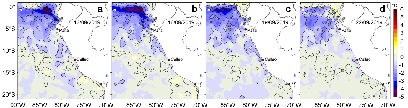
Figura 3. Anomalías de la temperatura superficial del mar (TSM, °C) para los días: a) 13, b) 16, c) 19 y d) 22 de setiembre de 2019. Las anomalías se calcularon respecto de la climatología para el periodo 2007-2016. Datos: OSTIA-UKMO-L4-GLOB-v2.0 (UK Met Office, 2012; Donlon et al, 2012). Procesamiento: LHF/AFIOF/DGIOCC/IMARPE.
