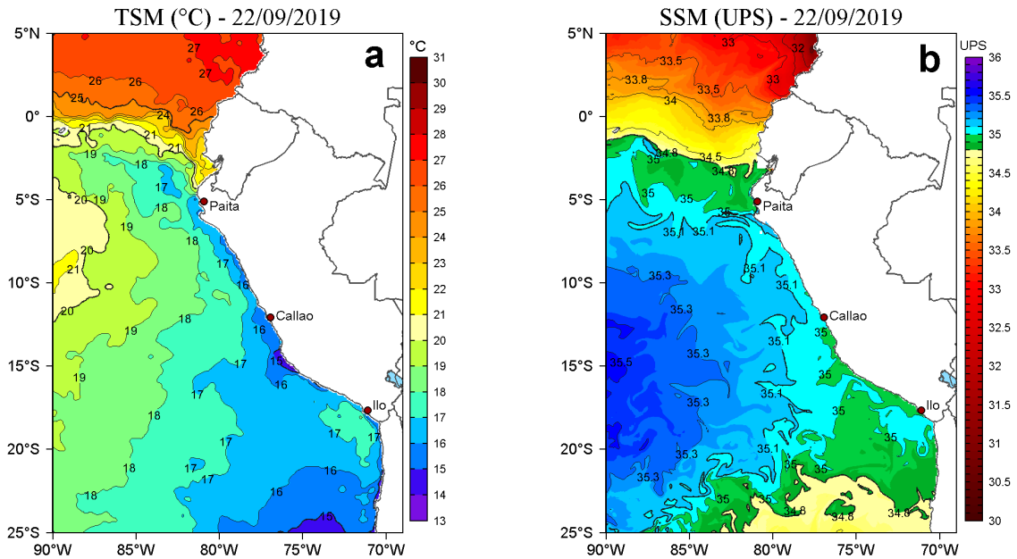
Figura 2. a) Temperatura superficial del mar (TSM, °C) y b) Salinidad superficial del mar (SSM, UPS), para el 22 de setiembre de 2019. Datos: OSTIA-UKMO-L4-GLOB-v2.0 (UK Met Office, 2012; Donlon et al, 2012) disponible en https://podaac.jpl.nasa.gov/dataset/OSTIA-UKMO-L4-GLOB-v2.0 para (a) y Hybrid Coordinate Ocean Model v. GOFS 3.1 (HYCOM; Halliwell et al., 1998; 2000; Bleck, 2001) para (b). Procesamiento: LHF/AFIOF/DGIOCC/IMARPE.
