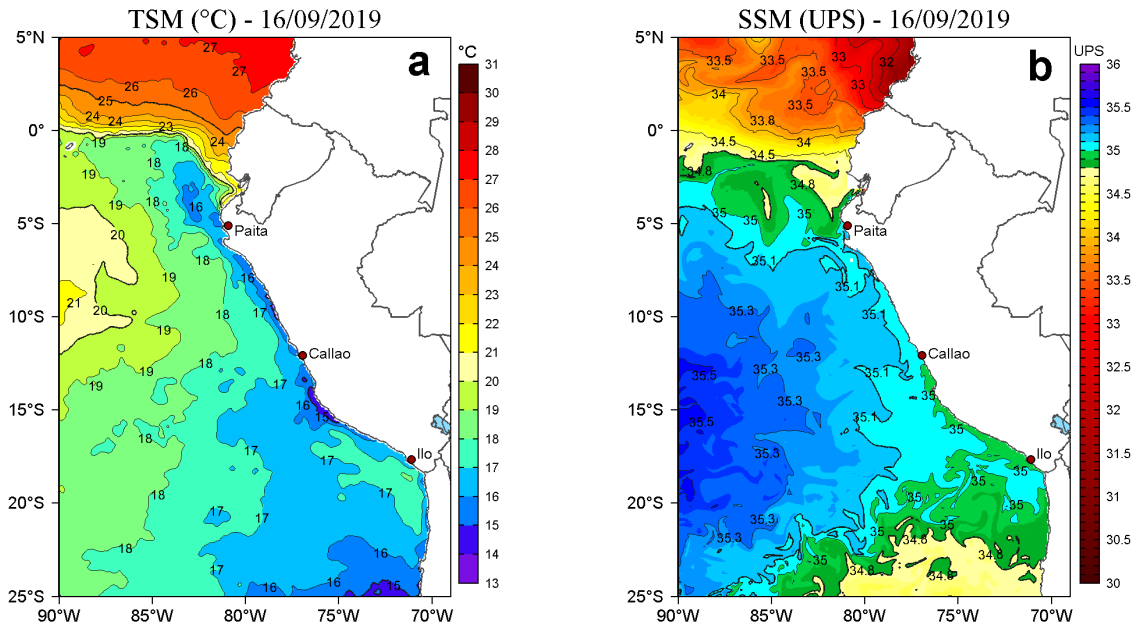
Figura 2. a) Temperatura superficial del mar (TSM, °C) y b) Salinidad superficial del mar (SSM, UPS), para el 16 de setiembre de 2019. Datos: OSTIA-UKMO-L4-GLOB-v2.0 (UK Met Office, 2012; Donlon et al, 2012) disponible en https://podaac.jpl.nasa.gov/dataset/OSTIA-UKMO-L4-GLOB-v2.0 para (a) y Hybrid Coordinate Ocean Model v. GOFS 3.1 (HYCOM; Halliwell et al., 1998; 2000; Bleck, 2001) para (b). Procesamiento: LHF/AFIOF/DGIOCC/IMARPE.
