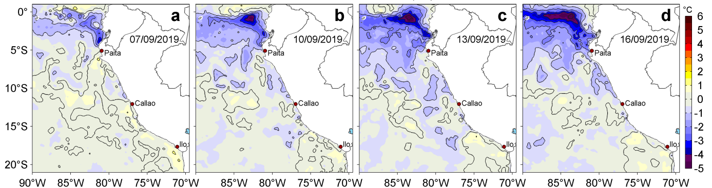
Figura 3. Anomalías de la temperatura superficial del mar (TSM, °C) para los días: a) 07, b) 10, c) 13 y d) 16 de setiembre de 2019. Las anomalías se calcularon respecto de la climatología para el periodo 2007-2016. Datos: OSTIA-UKMO-L4-GLOB-v2.0 (UK Met Office, 2012; Donlon et al, 2012). Procesamiento: LHF/AFIOF/DGIOCC/IMARPE.
