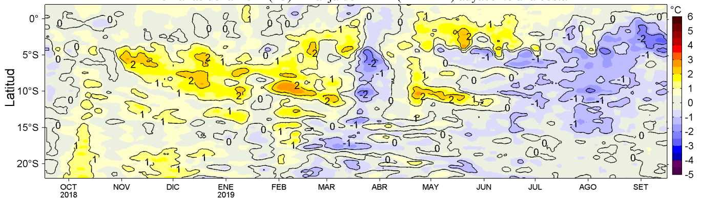
Figura 4. Variación promedio de las anomalías de la temperatura superficial del mar (TSM, °C) para una franja de 60 mn (~111 km) adyacente al litoral peruano para los últimos doce meses al 16 de setiembre de 2019. Datos: OSTIA-UKMO-L4-GLOB-v2.0 (UK Met. Office, 2012; Donlon et al, 2012) disponible en https://podaac.jpl.nasa.gov/dataset/OSTIA-UKMO-L4-GLOB-v2.0 . Las anomalías se calcularon con respecto al periodo 2007-2016. Procesamiento: LHF/AFIOF/DGIOCC/IMARPE.
