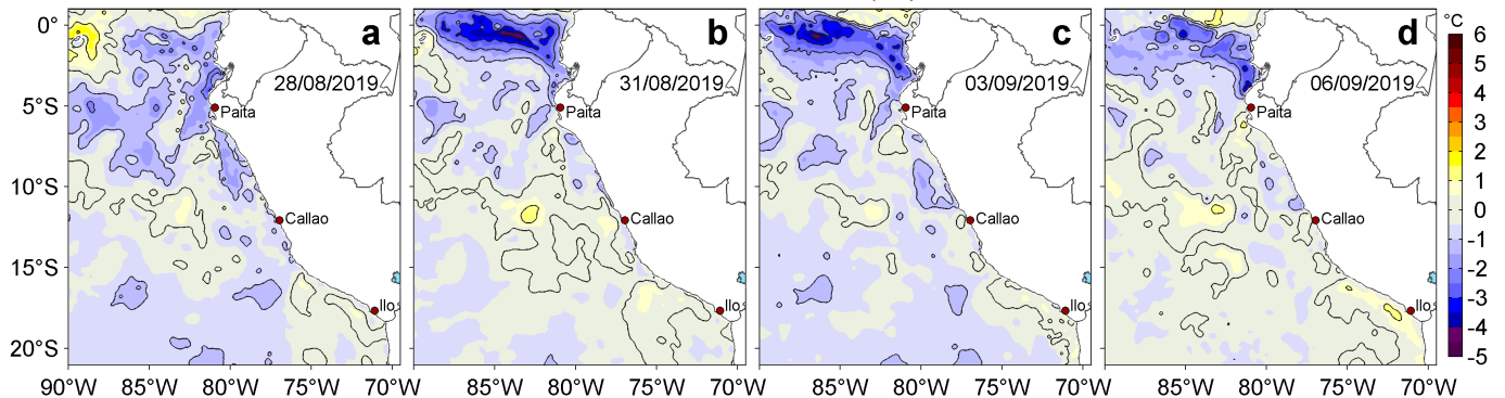
Figura 3. Anomalías de la temperatura superficial del mar (TSM, °C) para los días: a) 28 y b) 31 de agosto, c) 03 y d) 06 de setiembre de 2019. Las anomalías se calcularon respecto de la climatología para el periodo 2007-2016. Datos: OSTIA-UKMO-L4-GLOB-v2.0 (UK Met Office, 2012; Donlon et al, 2012). Procesamiento: LHF/AFIOF/DGIOCC/IMARPE.
