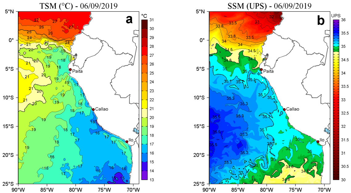
Figura 2. a) Temperatura superficial del mar (TSM, °C) y b) Salinidad superficial del mar (SSM, UPS), para el 06 de setiembre de 2019. Datos: OSTIA-UKMO-L4-GLOB-v2.0 (UK Met Office, 2012; Donlon et al, 2012) disponible en https://podaac.jpl.nasa.gov/dataset/OSTIA-UKMO-L4-GLOB-v2.0 para (a) y Hybrid Coordinate Ocean Model v. GOFS 3.1 (HYCOM; Halliwell et al., 1998; 2000; Bleck, 2001) para (b). Procesamiento: LHF/AFIOF/DGIOCC/IMARPE.
