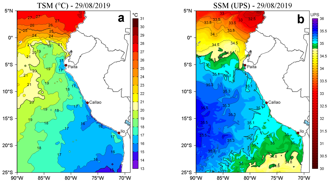
Figura 2. a) Temperatura superficial del mar (TSM, °C) y b) Salinidad superficial del mar (SSM, UPS), para el 29 de agosto de 2019. Datos: OSTIA-UKMO-L4-GLOB-v2.0 (UK Met Office, 2012; Donlon et al, 2012) disponible en https://podaac.jpl.nasa.gov/dataset/OSTIA-UKMO-L4-GLOB-v2.0 para (a) y Hybrid Coordinate Ocean Model v. GOFs 3.1 (HYCOM; Halliwell et al., 1998; 2000; Bleck, 2001) para (b). Procesamiento: LHF/AFIOF/DGIOCC/IMARPE.
