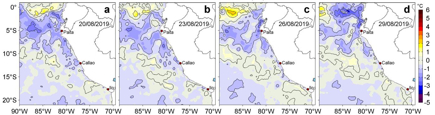
Figura 3. Anomalías de la temperatura superficial del mar (TSM, °C) para los días: a) 20, b) 23, c) 26 y d) 29 de agosto de 2019. Las anomalías se calcularon respecto de la climatología para el periodo 2007-2016. Datos: OSTIA-UKMO-L4-GLOB-v2.0 (UK Met Office, 2012; Donlon et al, 2012). Procesamiento: LHF/AFIOF/DGIOCC/IMARPE.
