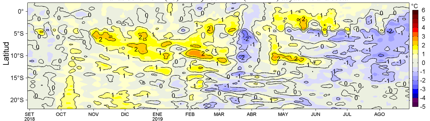
Figura 4. Variación promedio de las anomalías de la temperatura superficial del mar (TSM, °C) para una franja de 60 mn (~111 km) adyacente al litoral peruano para los últimos doce meses al 29 de agosto de 2019. Datos: OSTIA-UKMO-L4-GLOB-v2.0 (UK Met. Office, 2012; Donlon et al, 2012) disponible en https://podaac.jpl.nasa.gov/dataset/OSTIA-UKMO-L4-GLOB-v2.0 . Las anomalías se calcularon con respecto al periodo 2007-2016. Procesamiento: LHF/AFIOF/DGIOCC/IMARPE.
