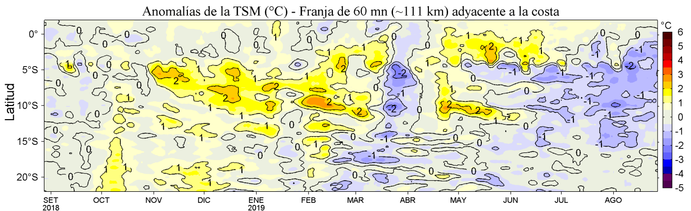
Figura 4. Variación promedio de las anomalías de la temperatura superficial del mar (TSM, °C) para una franja de 60 mn (~111 km) adyacente al litoral peruano para los últimos doce meses al 27 de agosto de 2019. Datos: OSTIA-UKMO-L4-GLOB-v2.0 (UK Met. Office, 2012; Donlon et al, 2012) disponible en https://podaac.jpl.nasa.gov/dataset/OSTIA-UKMO-L4-GLOB-v2.0 . Las anomalías se calcularon con respecto al periodo 2007-2016. Procesamiento: LHF/AFIOF/DGIOCC/IMARPE.
