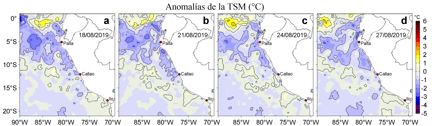
Figura 3. Anomalías de la temperatura superficial del mar (TSM, °C) para los días: a) 18, b) 21, c) 24 y d) 27 de agosto de 2019. Las anomalías se calcularon respecto de la climatología para el periodo 2007-2016. Datos: OSTIA-UKMO-L4-GLOB-v2.0 (UK Met Office, 2012; Donlon et al, 2012). Procesamiento: LHF/AFIOF/DGIOCC/IMARPE.
