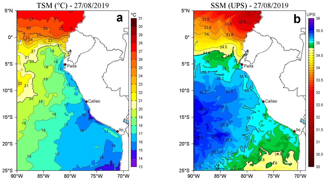
Figura 2. a) Temperatura superficial del mar (TSM, °C) y b) Salinidad superficial del mar (SSM, UPS), para el 27 de agosto de 2019. Datos: OSTIA-UKMO-L4-GLOB-v2.0 (UK Met Office, 2012; Donlon et al, 2012) disponible en https://podaac.jpl.nasa.gov/dataset/OSTIA-UKMO-L4-GLOB-v2.0 para (a) y Hybrid Coordinate Ocean Model v. GOF3.1 (HYCOM; Halliwell et al., 1998; 2000; Bleck, 2001) para (b). Procesamiento: LHF/AFIOF/DGIOCC/IMARPE.
