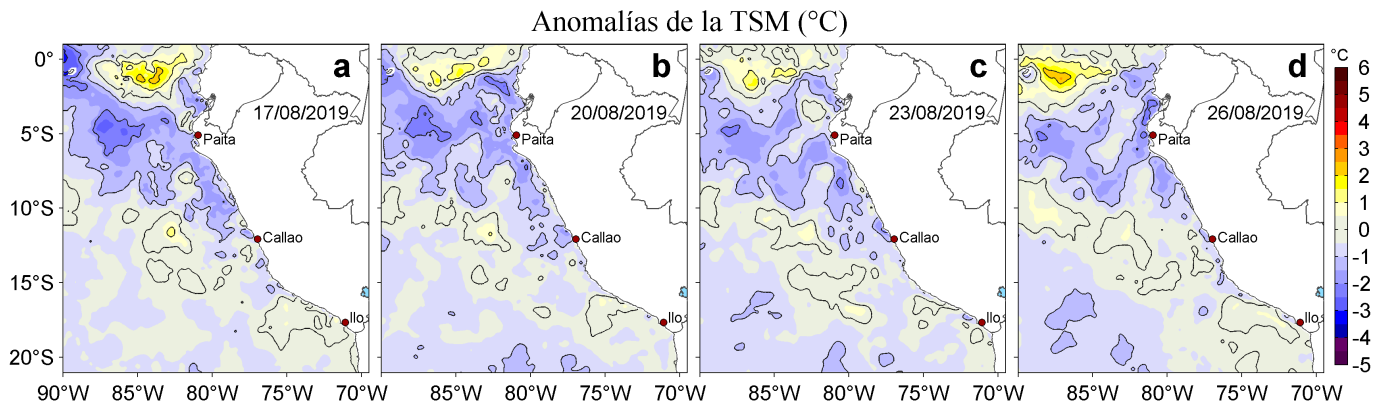
Figura 3. Anomalías de la temperatura superficial del mar (TSM, °C) para los días: a) 17, b) 20, c) 23 y d) 26 de agosto de 2019. Las anomalías se calcularon respecto de la climatología para el periodo 2007-2016. Datos: OSTIA-UKMO-L4-GLOB-v2.0 (UK Met Office, 2012; Donlon et al, 2012). Procesamiento: LHF/AFIOF/DGIOCC/IMARPE.
