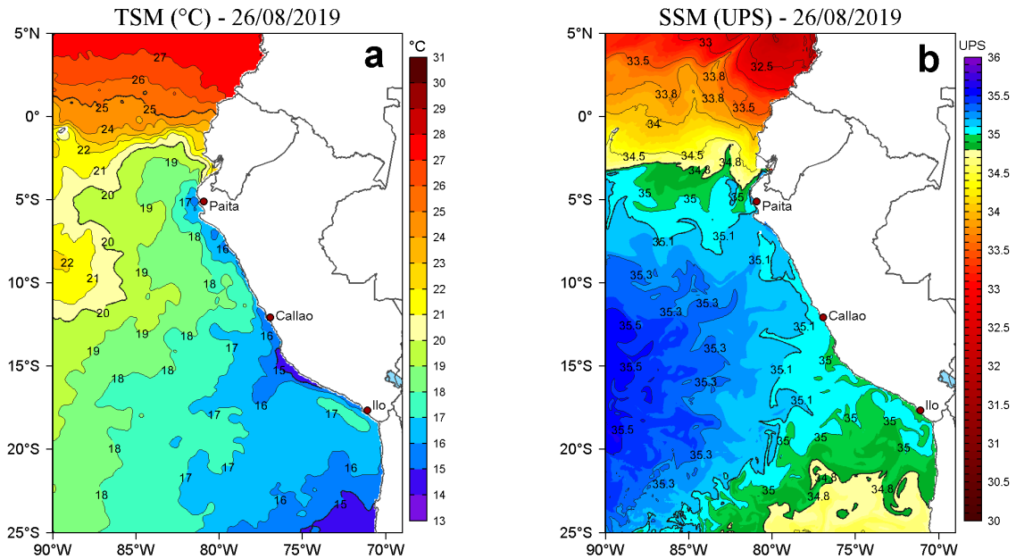
Figura 2. a) Temperatura superficial del mar (TSM, °C) y b) Salinidad superficial del mar (SSM, UPS), para el 26 de agosto de 2019. Datos: OSTIA-UKMO-L4-GLOB-v2.0 (UK Met Office, 2012; Donlon et al, 2012) disponible en https://podaac.jpl.nasa.gov/dataset/OSTIA-UKMO-L4-GLOB-v2.0 para (a) y Hybrid Coordinate Ocean Model v. GOF3.1 (HYCOM; Halliwell et al., 1998; 2000; Bleck, 2001) para (b). Procesamiento: LHF/AFIOF/DGIOCC/IMARPE.
