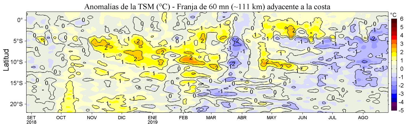
Figura 4. Variación promedio de las anomalías de la temperatura superficial del mar (TSM, °C) para una franja de 60 mn (~111 km) adyacente al litoral peruano para los últimos doce meses al 26 de agosto de 2019. Datos: OSTIA-UKMO-L4-GLOB-v2.0 (UK Met. Office, 2012; Donlon et al, 2012) disponible en https://podaac.jpl.nasa.gov/dataset/OSTIA-UKMO-L4-GLOB-v2.0 . Las anomalías se calcularon con respecto al periodo 2007-2016. Procesamiento: LHF/AFIOF/DGIOCC/IMARPE.
