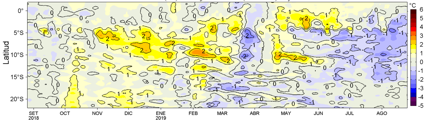
Figura 4. Variación promedio de las anomalías de la temperatura superficial del mar (TSM, °C) para una franja de 60 mn (~111 km) adyacente al litoral peruano para los últimos doce meses al 25 de agosto de 2019. Datos: OSTIA-UKMO-L4-GLOB-v2.0 (UK Met. Office, 2012; Donlon et al, 2012) disponible en https://podaac.jpl.nasa.gov/dataset/OSTIA-UKMO-L4-GLOB-v2.0 . Las anomalías se calcularon con respecto al periodo 2007-2016. Procesamiento: LHF/AFIOF/DGIOCC/IMARPE.
