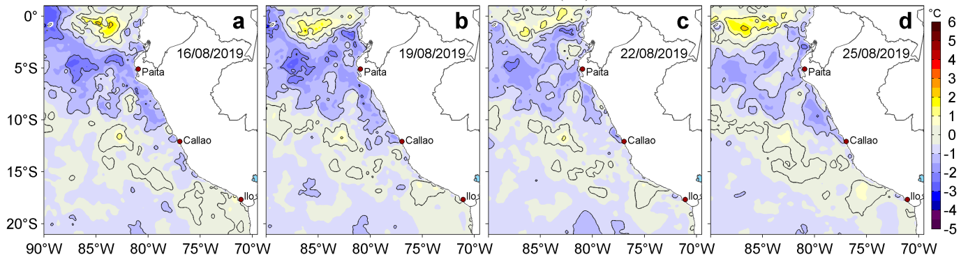
Figura 3. Anomalías de la temperatura superficial del mar (TSM, °C) para los días: a) 16, b) 19, c) 22 y d) 25 de agosto de 2019. Las anomalías se calcularon respecto de la climatología para el periodo 2007-2016. Datos: OSTIA-UKMO-L4-GLOB-v2.0 (UK Met Office, 2012; Donlon et al, 2012). Procesamiento: LHF/AFIOF/DGIOCC/IMARPE.
