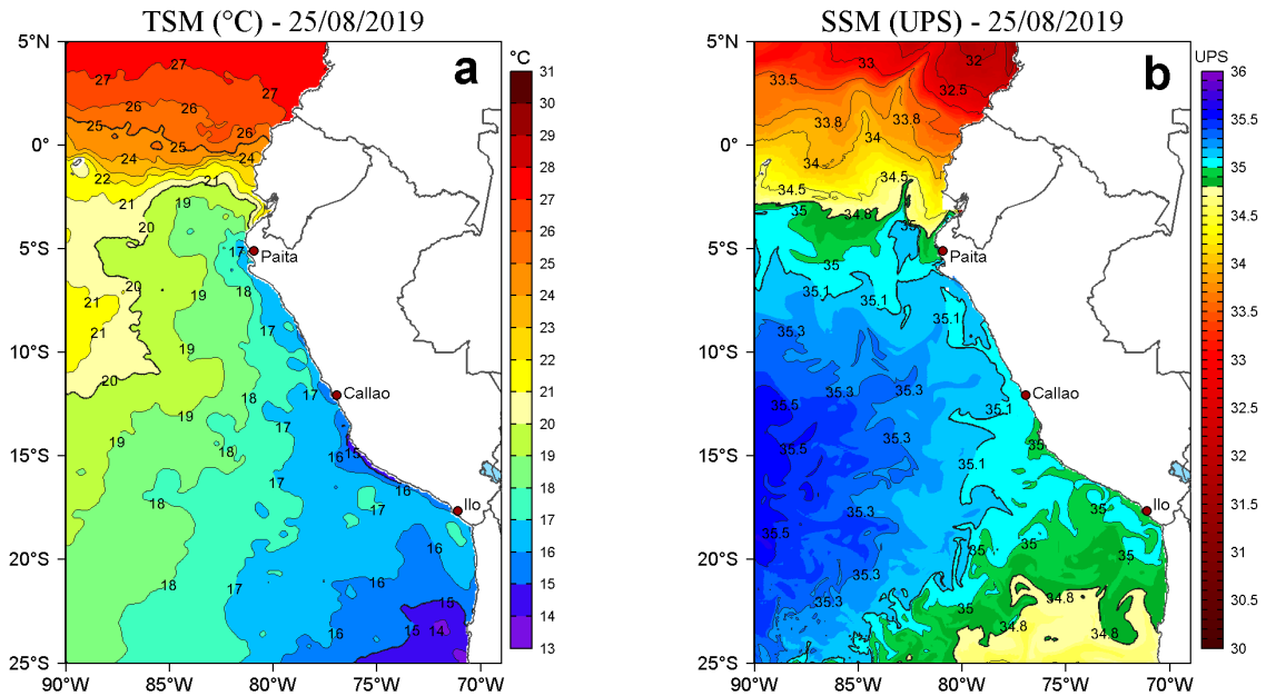
Figura 2. a) Temperatura superficial del mar (TSM, °C) y b) Salinidad superficial del mar (SSM, UPS), para el 25 de agosto de 2019. Datos: OSTIA-UKMO-L4-GLOB-v2.0 (UK Met Office, 2012; Donlon et al, 2012) disponible en https://podaac.jpl.nasa.gov/dataset/OSTIA-UKMO-L4-GLOB-v2.0 para (a) y Hybrid Coordinate Ocean Model v. GOF3 3.1 (HYCOM; Halliwell et al., 1998; 2000; Bleck, 2001) para (b). Procesamiento: LHF/AFIOF/DGIOCC/IMARPE.
