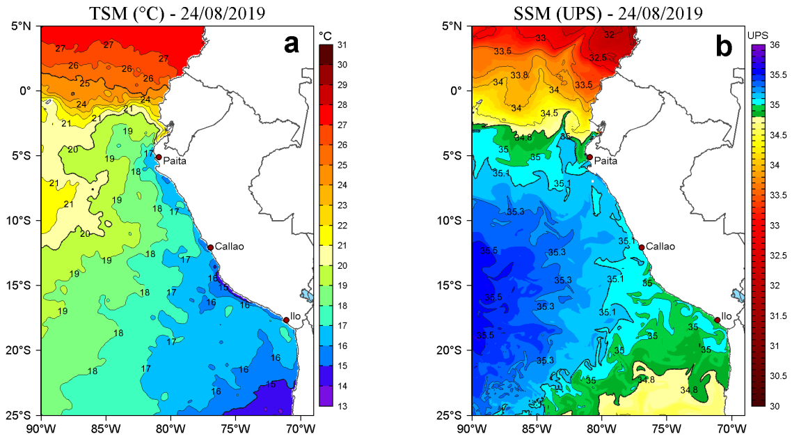
Figura 2. a) Temperatura superficial del mar (TSM, °C) y b) Salinidad superficial del mar (SSM, UPS), para el 24 de agosto de 2019. Datos: OSTIA-UKMO-L4-GLOB-v2.0 (UK Met Office, 2012; Donlon et al, 2012) disponible en https://podaac.jpl.nasa.gov/dataset/OSTIA-UKMO-L4-GLOB-v2.0 para (a) y Hybrid Coordinate Ocean Model v. GOF3 3.1 (HYCOM; Halliwell et al., 1998; 2000; Bleck, 2001) para (b). Procesamiento: LHF/AFIOF/DGIOCC/IMARPE.
