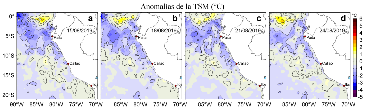
Figura 3. Anomalías de la temperatura superficial del mar (TSM, °C) para los días: a) 15, b) 18, c) 21 y d) 24 de agosto de 2019. Las anomalías se calcularon respecto de la climatología para el periodo 2007-2016. Datos: OSTIA-UKMO-L4-GLOB-v2.0 (UK Met Office, 2012; Donlon et al, 2012). Procesamiento: LHF/AFIOF/DGIOCC/IMARPE.
