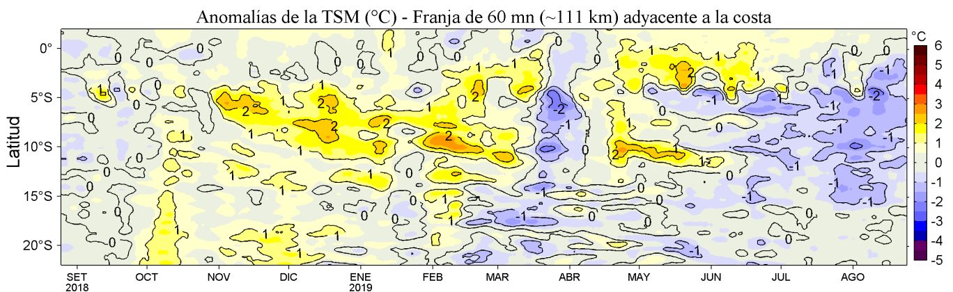
Figura 4. Variación promedio de las anomalías de la temperatura superficial del mar (TSM, °C) para una franja de 60 mn (~111 km) adyacente al litoral peruano para los últimos doce meses al 24 de agosto de 2019. Datos: OSTIA-UKMO-L4-GLOB-v2.0 (UK Met. Office, 2012; Donlon et al, 2012) disponible en https://podaac.jpl.nasa.gov/dataset/OSTIA-UKMO-L4-GLOB-v2.0 . Las anomalías se calcularon con respecto al periodo 2007-2016. Procesamiento: LHF/AFIOF/DGIOCC/IMARPE.
