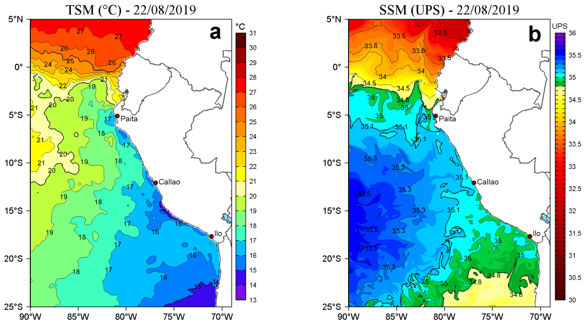
Figura 2. a) Temperatura superficial del mar (TSM, °C) y b) Salinidad superficial del mar (SSM, UPS), para el 22 de agosto de 2019. Datos: OSTIA-UKMO-L4-GLOB-v2.0 (UK Met Office, 2012; Donlon et al, 2012) disponible en https://podaac.jpl.nasa.gov/dataset/OSTIA-UKMO-L4-GLOB-v2.0 para (a) y Hybrid Coordinate Ocean Model v. GOF3 3.1 (HYCOM; Halliwell et al., 1998; 2000; Bleck, 2001) para (b). Procesamiento: LHF/AFIOF/DGIOCC/IMARPE.
