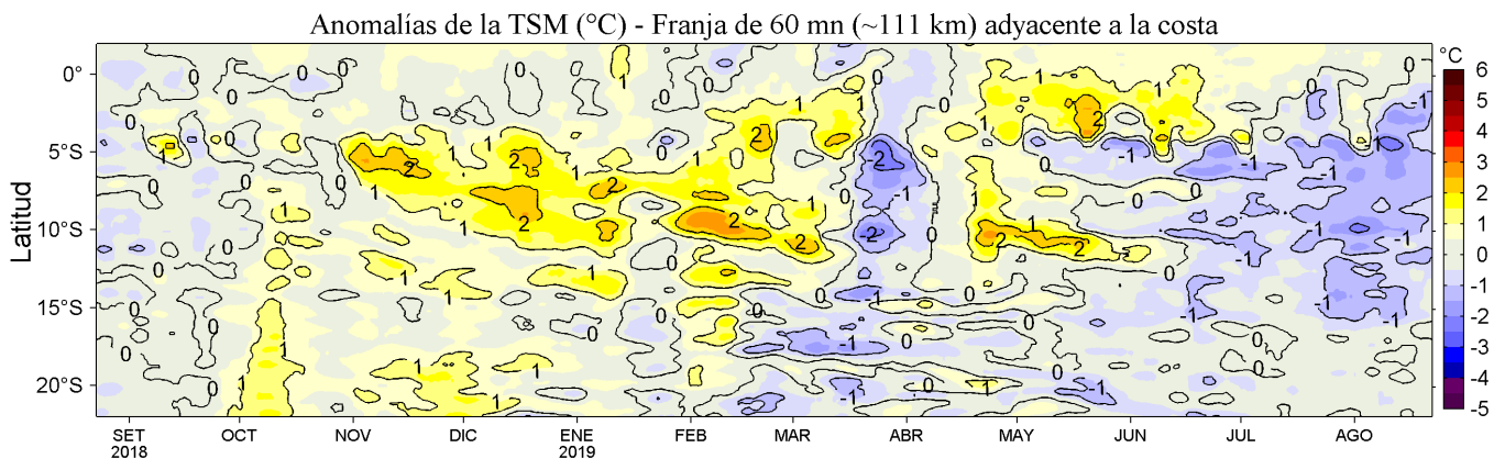
Figura 4. Variación promedio de las anomalías de la temperatura superficial del mar (TSM, °C) para una franja de 60 mn (~111 km) adyacente al litoral peruano para los últimos doce meses al 22 de agosto de 2019. Datos: OSTIA-UKMO-L4-GLOB-v2.0 (UK Met. Office, 2012; Donlon et al, 2012) disponible en https://podaac.jpl.nasa.gov/dataset/OSTIA-UKMO-L4-GLOB-v2.0 . Las anomalías se calcularon con respecto al periodo 2007-2016. Procesamiento: LHF/AFIOF/DGIOCC/IMARPE.
