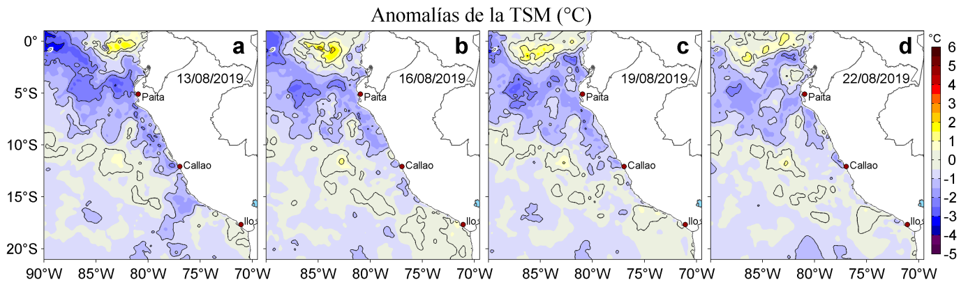
Figura 3. Anomalías de la temperatura superficial del mar (TSM, °C) para los días: a) 13, b) 16, c) 19 y d) 22 de agosto de 2019. Las anomalías se calcularon respecto de la climatología para el periodo 2007-2016. Datos: OSTIA-UKMO-L4-GLOB-v2.0 (UK Met Office, 2012; Donlon et al, 2012). Procesamiento: LHF/AFIOF/DGIOCC/IMARPE.
