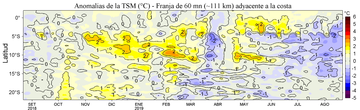
Figura 4. Variación promedio de las anomalías de la temperatura superficial del mar (TSM, °C) para una franja de 60 mn (~111 km) adyacente al litoral peruano para los últimos doce meses al 21 de agosto de 2019. Datos: OSTIA-UKMO-L4-GLOB-v2.0 (UK Met. Office, 2012; Donlon et al, 2012) disponible en https://podaac.jpl.nasa.gov/dataset/OSTIA-UKMO-L4-GLOB-v2.0 . Las anomalías se calcularon con respecto al periodo 2007-2016. Procesamiento: LHF/AFIOF/DGIOCC/IMARPE.
