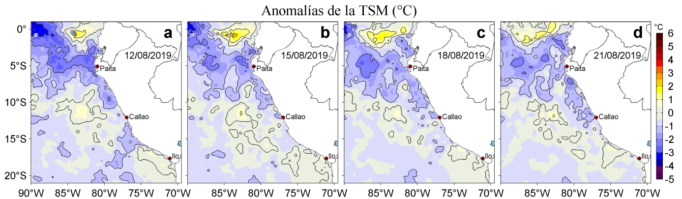
Figura 3. Anomalías de la temperatura superficial del mar (TSM, °C) para los días: a) 12, b) 15, c) 18 y d) 21 de agosto de 2019. Las anomalías se calcularon respecto de la climatología para el periodo 2007-2016. Datos: OSTIA-UKMO-L4-GLOB-v2.0 (UK Met Office, 2012; Donlon et al, 2012). Procesamiento: LHF/AFIOF/DGIOCC/IMARPE.
