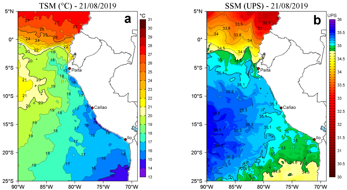
Figura 2. a) Temperatura superficial del mar (TSM, °C) y b) Salinidad superficial del mar (SSM, UPS), para el 21 de agosto de 2019. Datos: OSTIA-UKMO-L4-GLOB-v2.0 (UK Met Office, 2012; Donlon et al, 2012) disponible en https://podaac.jpl.nasa.gov/dataset/OSTIA-UKMO-L4-GLOB-v2.0 para (a) y Hybrid Coordinate Ocean Model v. GOF3 3.1 (HYCOM; Halliwell et al., 1998; 2000; Bleck, 2001) para (b). Procesamiento: LHF/AFIOF/DGIOCC/IMARPE.
