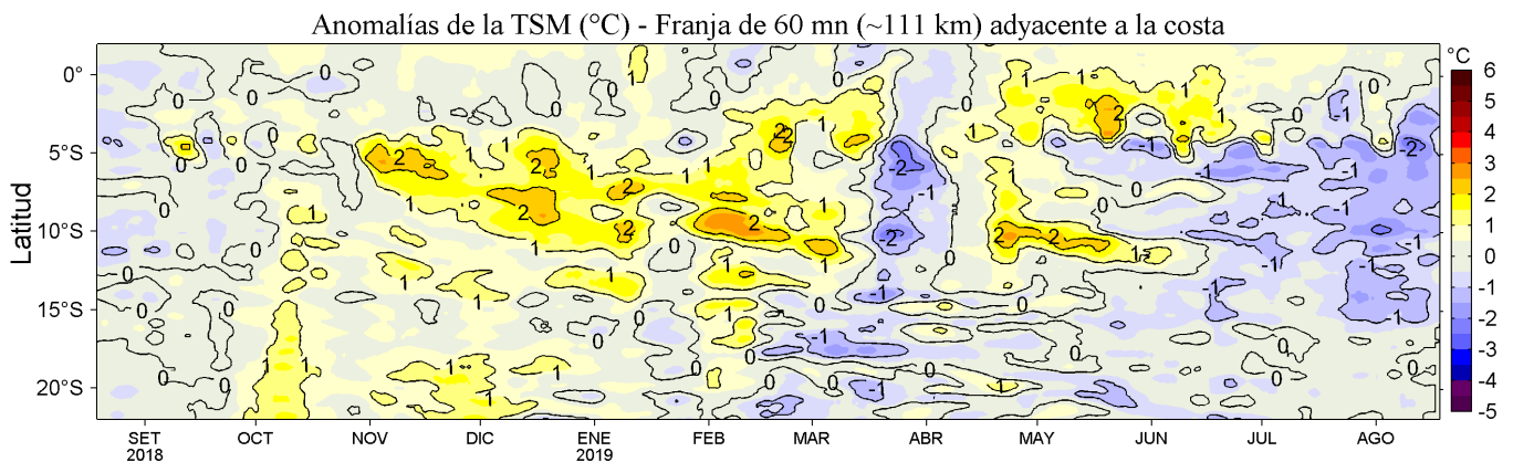
Figura 4. Variación promedio de las anomalías de la temperatura superficial del mar (TSM, °C) para una franja de 60 mn (~111 km) adyacente al litoral peruano para los últimos doce meses al 18 de agosto de 2019. Datos: OSTIA-UKMO-L4-GLOB-v2.0 (UK Met. Office, 2012; Donlon et al, 2012) disponible en https://podaac.jpl.nasa.gov/dataset/OSTIA-UKMO-L4-GLOB-v2.0 . Las anomalías se calcularon con respecto al periodo 2007-2016. Procesamiento: LHF/AFIOF/DGIOCC/IMARPE.
