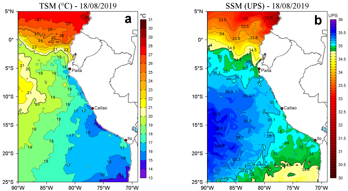
Figura 2. a) Temperatura superficial del mar (TSM, °C) y b) Salinidad superficial del mar (SSM, UPS), para el 18 de agosto de 2019. Datos: OSTIA-UKMO-L4-GLOB-v2.0 (UK Met Office, 2012; Donlon et al, 2012) disponible en https://podaac.jpl.nasa.gov/dataset/OSTIA-UKMO-L4-GLOB-v2.0 para (a) y Hybrid Coordinate Ocean Model v. GOF3 3.1 (HYCOM; Halliwell et al., 1998; 2000; Bleck, 2001) para (b). Procesamiento: LHF/AFIOF/DGIOCC/IMARPE.
