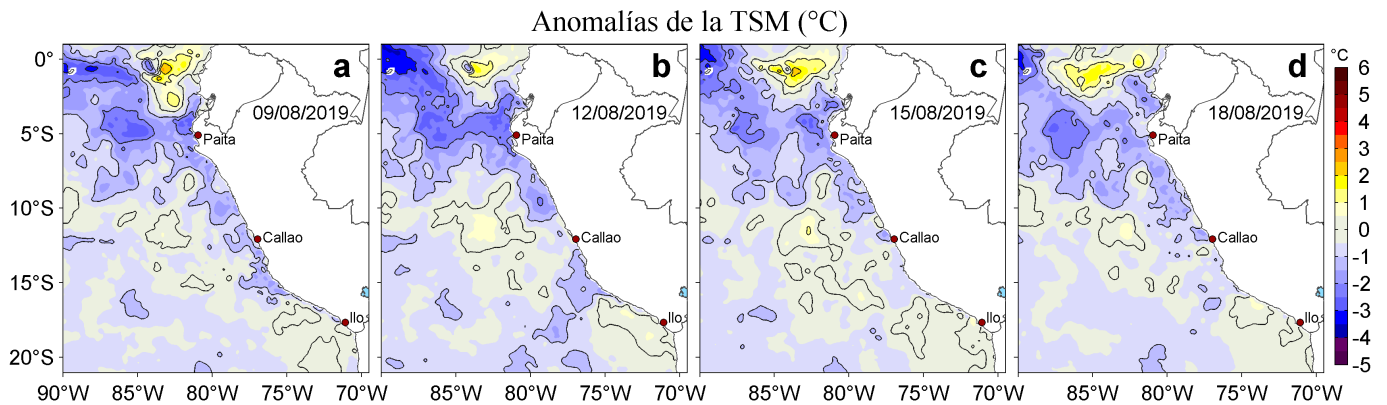
Figura 3. Anomalías de la temperatura superficial del mar (TSM, °C) para los días: a) 09, b) 12, c) 15 y d) 18 de agosto de 2019. Las anomalías se calcularon respecto de la climatología para el periodo 2007-2016. Datos: OSTIA-UKMO-L4-GLOB-v2.0 (UK Met Office, 2012; Donlon et al, 2012). Procesamiento: LHF/AFIOF/DGIOCC/IMARPE.
