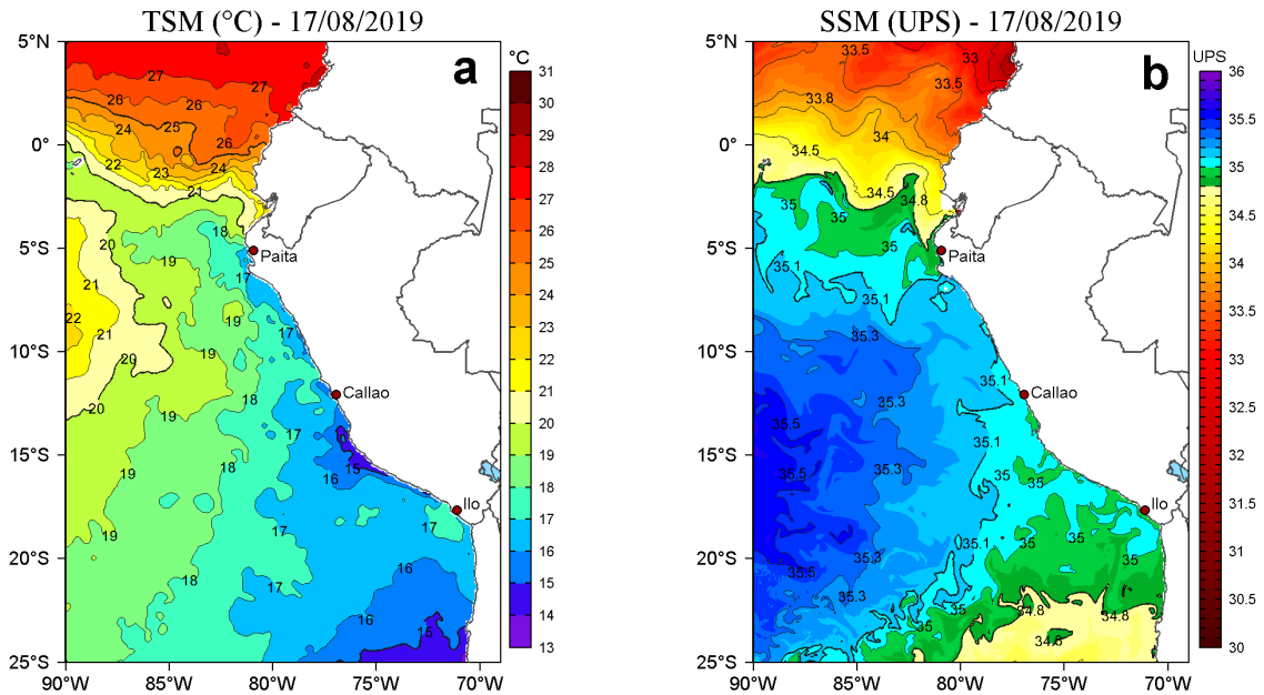
Figura 2. a) Temperatura superficial del mar (TSM, °C) y b) Salinidad superficial del mar (SSM, UPS), para el 17 de agosto de 2019. Datos: OSTIA-UKMO-L4-GLOB-v2.0 (UK Met Office, 2012; Donlon et al, 2012) disponible en https://podaac.jpl.nasa.gov/dataset/OSTIA-UKMO-L4-GLOB-v2.0 para (a) y Hybrid Coordinate Ocean Model v. GOF3 3.1 (HYCOM; Halliwell et al., 1998; 2000; Bleck, 2001) para (b). Procesamiento: LHF/AFIOF/DGIOCC/IMARPE.
