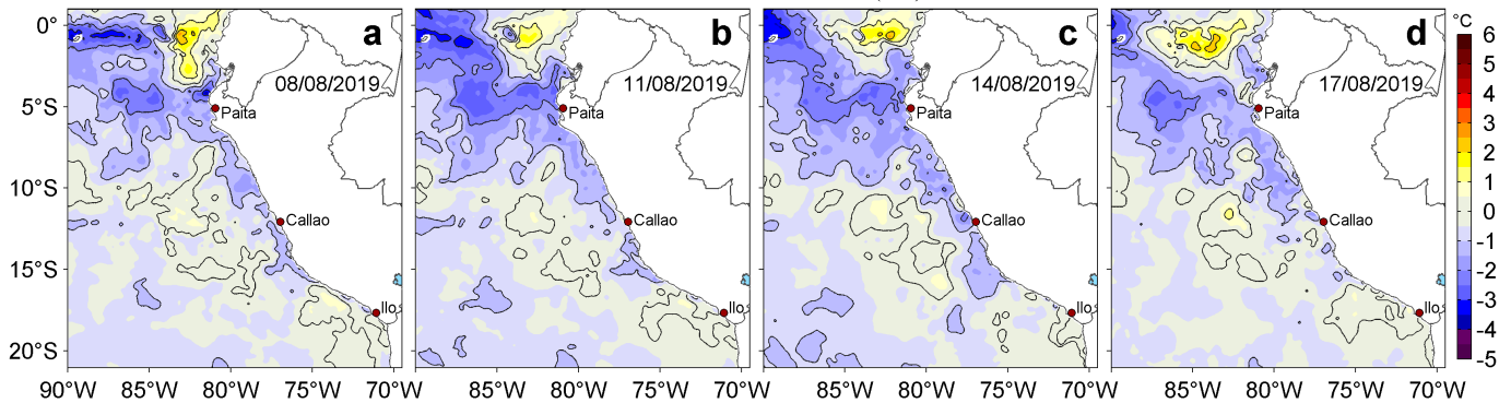
Figura 3. Anomalías de la temperatura superficial del mar (TSM, °C) para los días: a) 08, b) 11, c) 14 y d) 17 de agosto de 2019. Las anomalías se calcularon respecto de la climatología para el periodo 2007-2016. Datos: OSTIA-UKMO-L4-GLOB-v2.0 (UK Met Office, 2012; Donlon et al, 2012). Procesamiento: LHF/AFIOF/DGIOCC/IMARPE.
