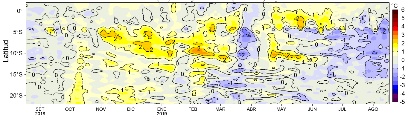
Figura 4. Variación promedio de las anomalías de la temperatura superficial del mar (TSM, °C) para una franja de 60 mn (~111 km) adyacente al litoral peruano para los últimos doce meses al 17 de agosto de 2019. Datos: OSTIA-UKMO-L4-GLOB-v2.0 (UK Met. Office, 2012; Donlon et al, 2012) disponible en https://podaac.jpl.nasa.gov/dataset/OSTIA-UKMO-L4-GLOB-v2.0 . Las anomalías se calcularon con respecto al periodo 2007-2016. Procesamiento: LHF/AFIOF/DGIOCC/IMARPE.
