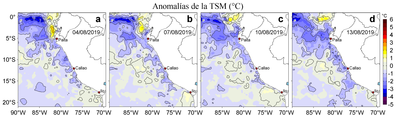
Figura 3. Anomalías de la temperatura superficial del mar (TSM, °C) para los días: a) 04, b) 07, c) 10 y d) 13 de agosto de 2019. Las anomalías se calcularon respecto de la climatología para el periodo 2007-2016. Datos: OSTIA-UKMO-L4-GLOB-v2.0 (UK Met Office, 2012; Donlon et al, 2012). Procesamiento: LHF/AFIOF/DGIOCC/IMARPE.
