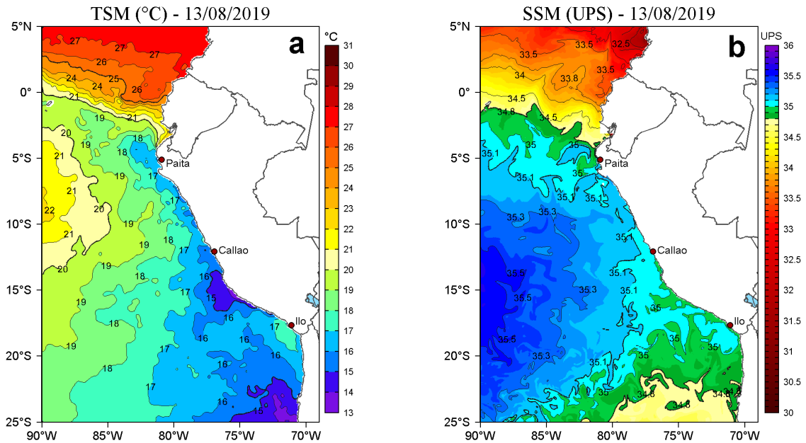
Figura 2. a) Temperatura superficial del mar (TSM, °C) y b) Salinidad superficial del mar (SSM, UPS), para el 13 de agosto de 2019. Datos: OSTIA-UKMO-L4-GLOB-v2.0 (UK Met Office, 2012; Donlon et al, 2012) disponible en https://podaac.jpl.nasa.gov/dataset/OSTIA-UKMO-L4-GLOB-v2.0 para (a) y Hybrid Coordinate Ocean Model v. GOF3 3.1 (HYCOM; Halliwell et al., 1998; 2000; Bleck, 2001) para (b). Procesamiento: LHF/AFIOF/DGIOCC/IMARPE.
