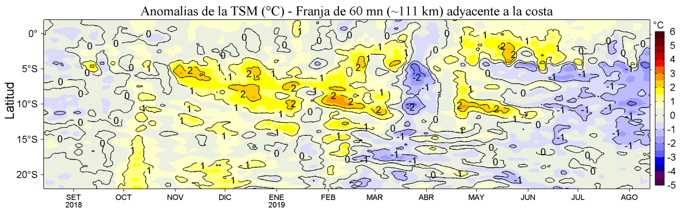
Figura 4. Variación promedio de las anomalías de la temperatura superficial del mar (TSM, °C) para una franja de 60 mn (~111 km) adyacente al litoral peruano para los últimos doce meses al 13 de agosto de 2019. Datos: OSTIA-UKMO-L4-GLOB-v2.0 (UK Met. Office, 2012; Donlon et al, 2012) disponible en https://podaac.jpl.nasa.gov/dataset/OSTIA-UKMO-L4-GLOB-v2.0 . Las anomalías se calcularon con respecto al periodo 2007-2016. Procesamiento: LHF/AFIOF/DGIOCC/IMARPE.
