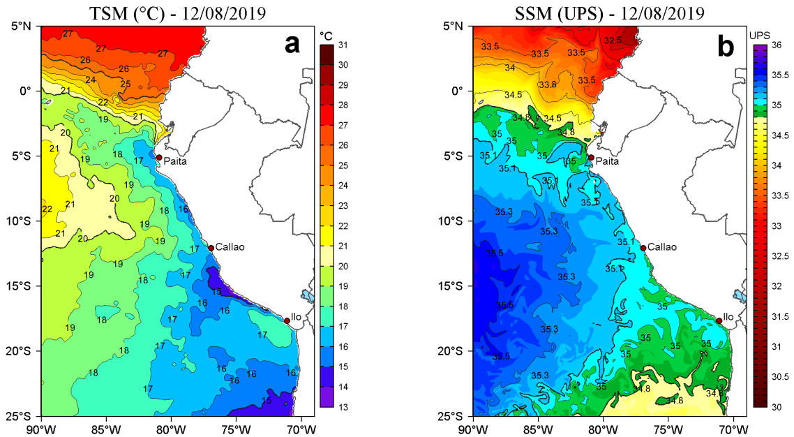
Figura 2. a) Temperatura superficial del mar (TSM, °C) y b) Salinidad superficial del mar (SSM, UPS), para el 12 de agosto de 2019. Datos: OSTIA-UKMO-L4-GLOB-v2.0 (UK Met Office, 2012; Donlon et al, 2012) disponible en https://podaac.jpl.nasa.gov/dataset/OSTIA-UKMO-L4-GLOB-v2.0 para (a) y Hybrid Coordinate Ocean Model v. GOF3 3.1 (HYCOM; Halliwell et al., 1998; 2000; Bleck, 2001) para (b). Procesamiento: LHF/AFIOF/DGIOCC/IMARPE.
