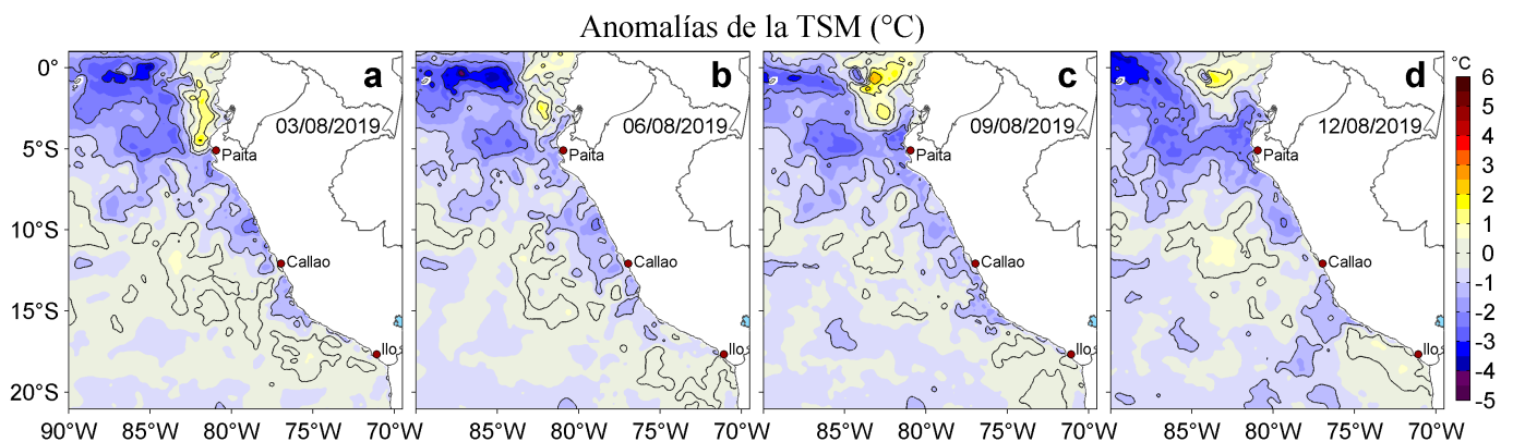
Figura 3. Anomalías de la temperatura superficial del mar (TSM, °C) para los días: a) 03, b) 06, c) 09 y d) 12 de agosto de 2019. Las anomalías se calcularon respecto de la climatología para el periodo 2007-2016. Datos: OSTIA-UKMO-L4-GLOB-v2.0 (UK Met Office, 2012; Donlon et al, 2012). Procesamiento: LHF/AFIOF/DGIOCC/IMARPE.
