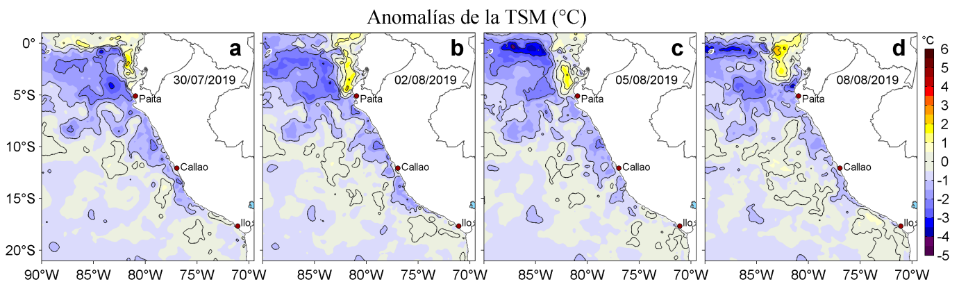
Figura 3. Anomalías de la temperatura superficial del mar (TSM, °C) para los días: a) 30 de julio, b) 02, c) 05 y d) 08 de agosto de 2019. Las anomalías se calcularon respecto de la climatología para el periodo 2007-2016. Datos: OSTIA-UKMO-L4-GLOB-v2.0 (UK Met Office, 2012; Donlon et al, 2012). Procesamiento: LHF/AFIOF/DGIOCC/IMARPE.
