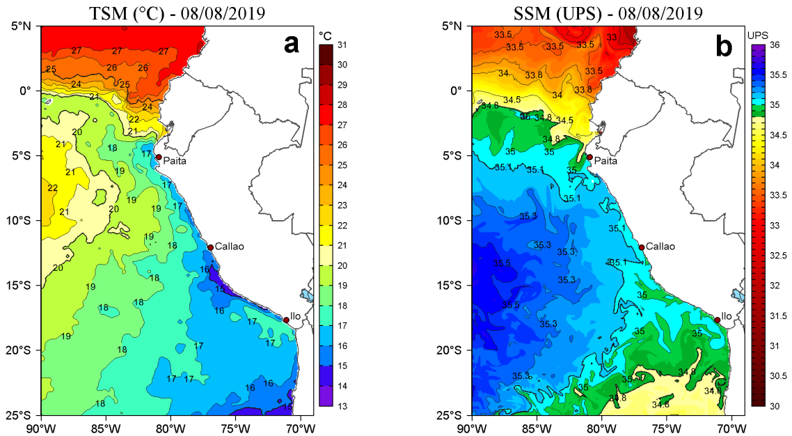
Figura 2. a) Temperatura superficial del mar (TSM, °C) y b) Salinidad superficial del mar (SSM, UPS), para el 08 de agosto de 2019. Datos: OSTIA-UKMO-L4-GLOB-v2.0 (UK Met Office, 2012; Donlon et al, 2012) disponible en https://podaac.jpl.nasa.gov/dataset/OSTIA-UKMO-L4-GLOB-v2.0 para (a) y Hybrid Coordinate Ocean Model v. GOF3 3.1 (HYCOM; Halliwell et al., 1998; 2000; Bleck, 2001) para (b). Procesamiento: LHF/AFIOF/DGIOCC/IMARPE.
