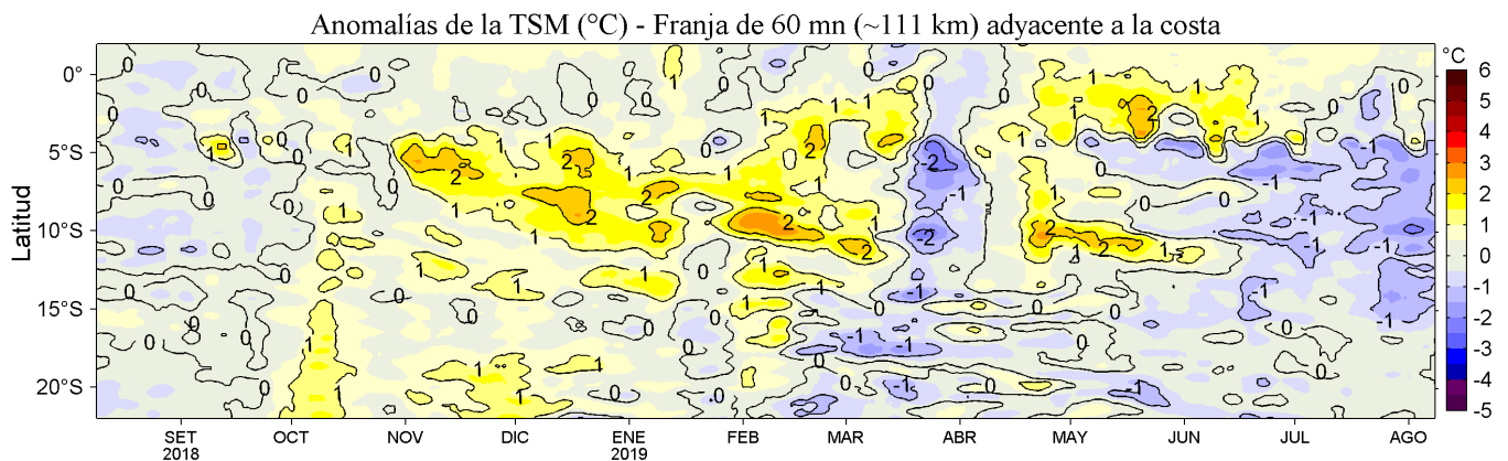
Figura 4. Variación promedio de las anomalías de la temperatura superficial del mar (TSM, °C) para una franja de 60 mn (~111 km) adyacente al litoral peruano para los últimos doce meses al 08 de agosto de 2019. Datos: OSTIA-UKMO-L4-GLOB-v2.0 (UK Met. Office, 2012; Donlon et al, 2012) disponible en https://podaac.jpl.nasa.gov/dataset/OSTIA-UKMO-L4-GLOB-v2.0 . Las anomalías se calcularon con respecto al periodo 2007-2016. Procesamiento: LHF/AFIOF/DGIOCC/IMARPE.
