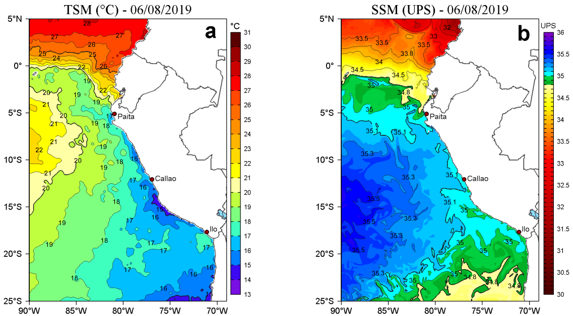
Figura 2. a) Temperatura superficial del mar (TSM, °C) y b) Salinidad superficial del mar (SSM, UPS), para el 06 de agosto de 2019. Datos: OSTIA-UKMO-L4-GLOB-v2.0 (UK Met Office, 2012; Donlon et al, 2012) disponible en https://podaac.jpl.nasa.gov/dataset/OSTIA-UKMO-L4-GLOB-v2.0 para (a) y Hybrid Coordinate Ocean Model v. GOF3 3.1 (HYCOM; Halliwell et al., 1998; 2000; Bleck, 2001) para (b). Procesamiento: LHF/AFIOF/DGIOCC/IMARPE.
