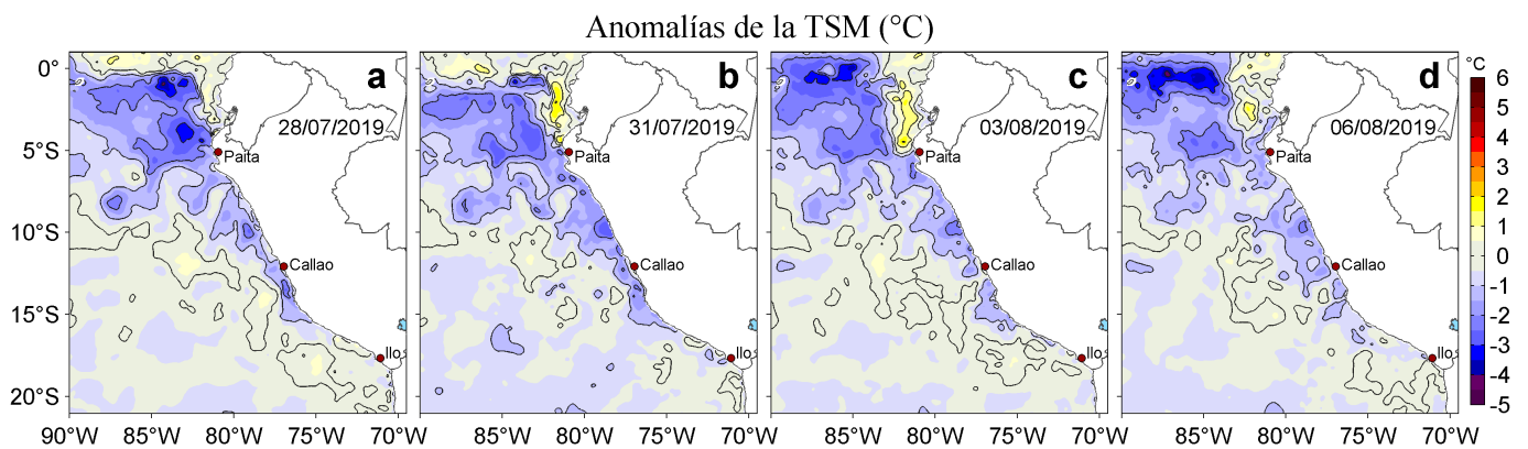
Figura 3. Anomalías de la temperatura superficial del mar (TSM, °C) para los días: a) 28 y b) 31 de julio, c) 03 y d) 06 de agosto de 2019. Las anomalías se calcularon respecto de la climatología para el periodo 2007-2016. Datos: OSTIA-UKMO-L4-GLOB-v2.0 (UK Met Office, 2012; Donlon et al, 2012). Procesamiento: LHF/AFIOF/DGIOCC/IMARPE.
