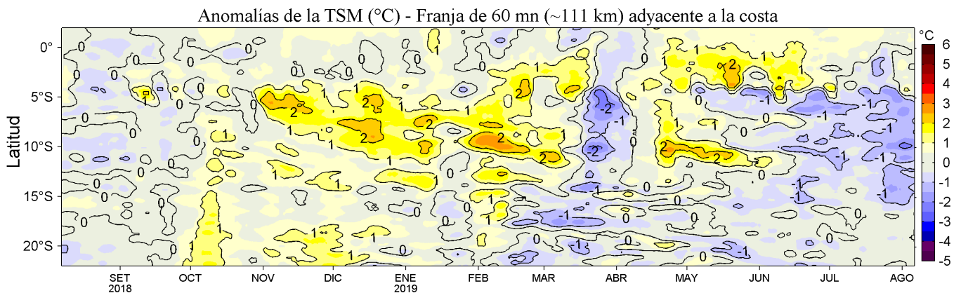
Figura 4. Variación promedio de las anomalías de la temperatura superficial del mar (TSM, °C) para una franja de 60 mn (~111 km) adyacente al litoral peruano para los últimos doce meses al 06 de agosto de 2019. Datos: OSTIA-UKMO-L4-GLOB-v2.0 (UK Met. Office, 2012; Donlon et al, 2012) disponible en https://podaac.jpl.nasa.gov/dataset/OSTIA-UKMO-L4-GLOB-v2.0 . Las anomalías se calcularon con respecto al periodo 2007-2016. Procesamiento: LHF/AFIOF/DGIOCC/IMARPE.
