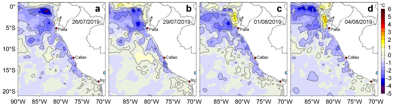
Figura 3. Anomalías de la temperatura superficial del mar (TSM, °C) para los días: a) 26 y b) 29 de julio, c) 01 y d) 04 de agosto de 2019. Las anomalías se calcularon respecto de la climatología para el periodo 2007-2016. Datos: OSTIA-UKMO-L4-GLOB-v2.0 (UK Met Office, 2012; Donlon et al, 2012). Procesamiento: LHF/AFIOF/DGIOCC/IMARPE.
