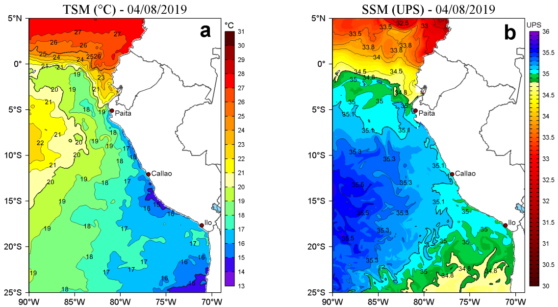
Figura 2. a) Temperatura superficial del mar (TSM, °C) y b) Salinidad superficial del mar (SSM, UPS), para el 04 de agosto de 2019. Datos: OSTIA-UKMO-L4-GLOB-v2.0 (UK Met Office, 2012; Donlon et al, 2012) disponible en https://podaac.jpl.nasa.gov/dataset/OSTIA-UKMO-L4-GLOB-v2.0 para (a) y Hybrid Coordinate Ocean Model v. GOF3 3.1 (HYCOM; Halliwell et al., 1998; 2000; Bleck, 2001) para (b). Procesamiento: LHF/AFIOF/DGIOCC/IMARPE.
