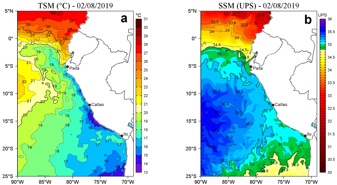
Figura 2. a) Temperatura superficial del mar (TSM, °C) y b) Salinidad superficial del mar (SSM, UPS), para el 02 de agosto de 2019. Datos: OSTIA-UKMO-L4-GLOB-v2.0 (UK Met Office, 2012; Donlon et al, 2012) disponible en https://podaac.jpl.nasa.gov/dataset/OSTIA-UKMO-L4-GLOB-v2.0 para (a) y Hybrid Coordinate Ocean Model v. GOF5 3.1 (HYCOM; Halliwell et al., 1998; 2000; Bleck, 2001) para (b). Procesamiento: LHF/AFIOF/DGIOCC/IMARPE.
