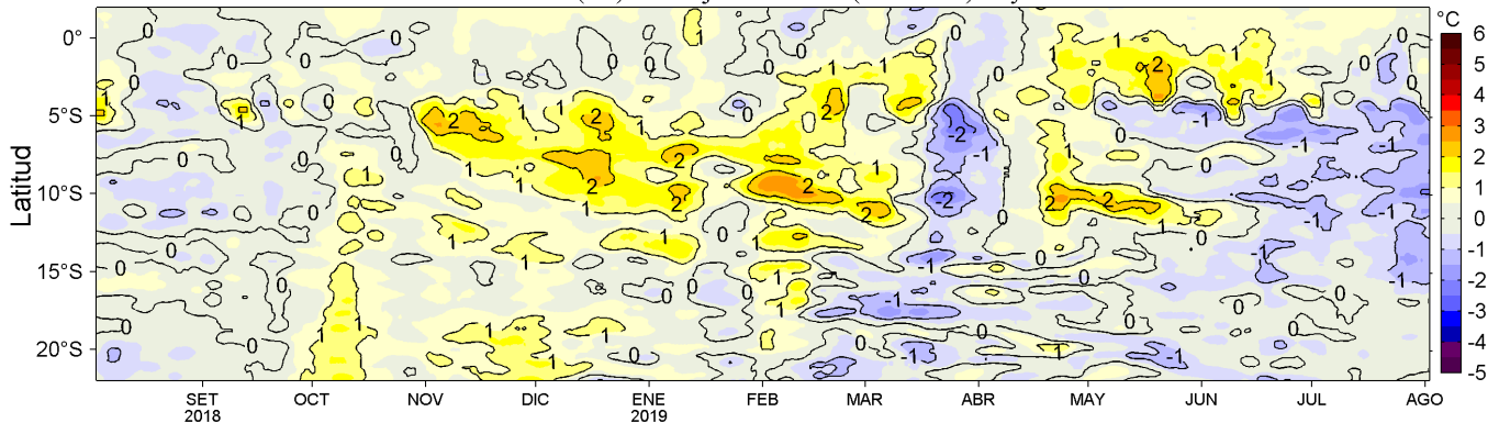
Figura 4. Variación promedio de las anomalías de la temperatura superficial del mar (TSM, °C) para una franja de 60 mn (~111 km) adyacente al litoral peruano para los últimos doce meses al 02 de agosto de 2019. Datos: OSTIA-UKMO-L4-GLOB-v2.0 (UK Met. Office, 2012; Donlon et al, 2012) disponible en https://podaac.jpl.nasa.gov/dataset/OSTIA-UKMO-L4-GLOB-v2.0 . Las anomalías se calcularon con respecto al periodo 2007-2016. Procesamiento: LHF/AFIOF/DGIOCC/IMARPE.
