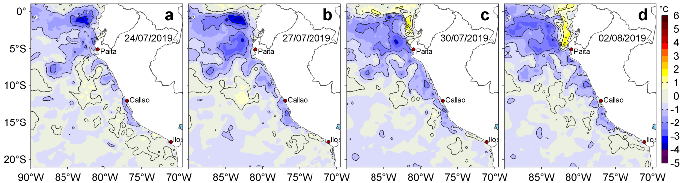
Figura 3. Anomalías de la temperatura superficial del mar (TSM, °C) para los días: a) 24, b) 27 y c) 30 de julio y d) 02 de agosto de 2019. Las anomalías se calcularon respecto de la climatología para el periodo 2007-2016. Datos: OSTIA-UKMO-L4-GLOB-v2.0 (UK Met Office, 2012; Donlon et al, 2012). Procesamiento: LHF/AFIOF/DGIOCC/IMARPE.
