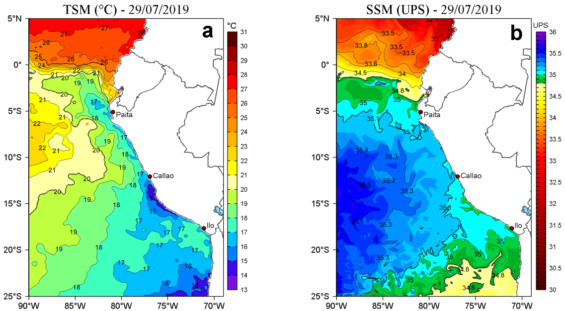
Figura 2. a) Temperatura superficial del mar (TSM, °C) y b) Salinidad superficial del mar (SSM, UPS), para el 29 de julio de 2019. Datos: OSTIA-UKMO-L4-GLOB-v2.0 (UK Met Office, 2012; Donlon et al, 2012) disponible en https://podaac.jpl.nasa.gov/dataset/OSTIA-UKMO-L4-GLOB-v2.0 para (a) y Hybrid Coordinate Ocean Model v. GOFs 3.1 (HYCOM; Halliwell et al., 1998; 2000; Bleck, 2001) para (b). Procesamiento: LHFM/AFIOF/DGIOCC/IMARPE.
