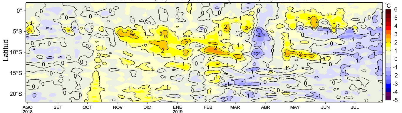
Figura 4. Variación promedio de las anomalías de la temperatura superficial del mar (TSM, °C) para una franja de 60 mn (~111 km) adyacente al litoral peruano para los últimos doce meses al 29 de julio de 2019. Datos: OSTIA-UKMO-L4-GLOB-v2.0 (UK Met. Office, 2012; Donlon et al, 2012) disponible en https://podaac.jpl.nasa.gov/dataset/OSTIA-UKMO-L4-GLOB-v2.0 . Las anomalías se calcularon con respecto al periodo 2007-2016. Procesamiento: LHFM/AFIOF/DGIOCC/IMARPE.
