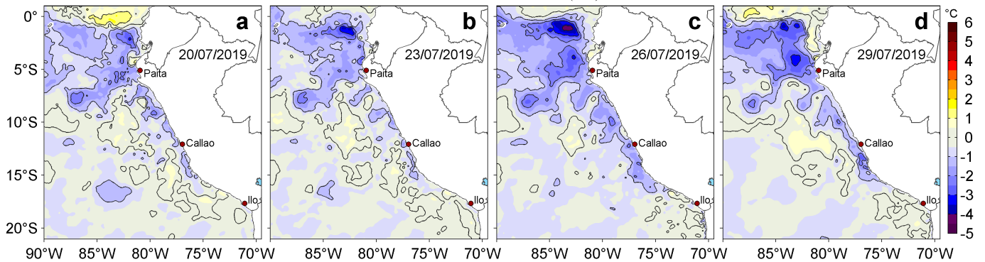
Figura 3. Anomalías de la temperatura superficial del mar (TSM, °C) para los días: a) 20, b) 23, c) 26 y d) 29 de julio de 2019. Las anomalías se calcularon respecto de la climatología para el periodo 2007-2016. Datos: OSTIA-UKMO-L4-GLOB-v2.0 (UK Met Office, 2012; Donlon et al, 2012). Procesamiento: LHFM/AFIOF/DGIOCC/IMARPE.
