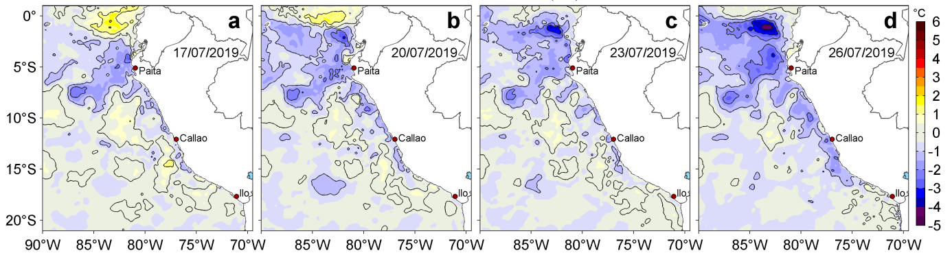
Figura 3. Anomalías de la temperatura superficial del mar (TSM, °C) para los días: a) 17, b) 20, c) 23 y d) 26 de julio de 2019. Las anomalías se calcularon respecto de la climatología para el periodo 2007-2016. Datos: OSTIA-UKMO-L4-GLOB-v2.0 (UK Met Office, 2012; Donlon et al, 2012). Procesamiento: LHFM/AFIOF/DGIOCC/IMARPE.
