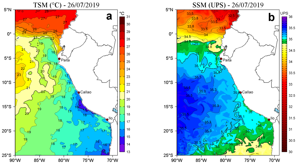
Figura 2. a) Temperatura superficial del mar (TSM, °C) y b) Salinidad superficial del mar (SSM, UPS), para el 26 de julio de 2019. Datos: OSTIA-UKMO-L4-GLOB-v2.0 (UK Met Office, 2012; Donlon et al, 2012) disponible en https://podaac.jpl.nasa.gov/dataset/OSTIA-UKMO-L4-GLOB-v2.0 para (a) y Hybrid Coordinate Ocean Model v. GOF3.1 (HYCOM; Halliwell et al., 1998; 2000; Bleck, 2001) para (b). Procesamiento: LHFM/AFIOF/DGIOCC/IMARPE.
