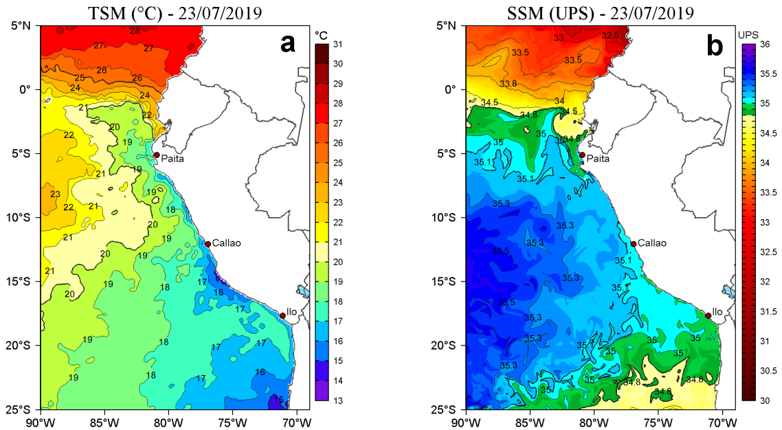
Figura 2. a) Temperatura superficial del mar (TSM, °C) y b) Salinidad superficial del mar (SSM, UPS), para el 23 de julio de 2019. Datos: OSTIA-UKMO-L4-GLOB-v2.0 (UK Met Office, 2012; Donlon et al, 2012) disponible en https://podaac.jpl.nasa.gov/dataset/OSTIA-UKMO-L4-GLOB-v2.0 para (a) y Hybrid Coordinate Ocean Model v. GOF5 3.1 (HYCOM; Halliwell et al., 1998; 2000; Bleck, 2001) para (b). Procesamiento: LHF/AFIOF/DGIOCC/IMARPE.
