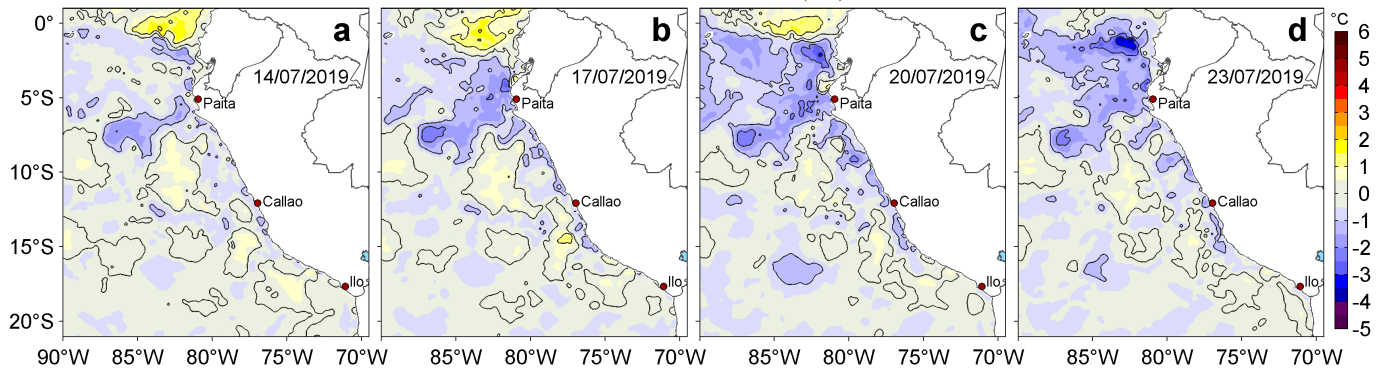
Figura 3. Anomalías de la temperatura superficial del mar (TSM, °C) para los días: a) 14, b) 17, c) 20 y d) 23 de julio de 2019. Las anomalías se calcularon respecto de la climatología para el periodo 2007-2016. Datos: OSTIA-UKMO-L4-GLOB-v2.0 (UK Met Office, 2012; Donlon et al, 2012). Procesamiento: LHF/AFIOF/DGIOCC/IMARPE.
