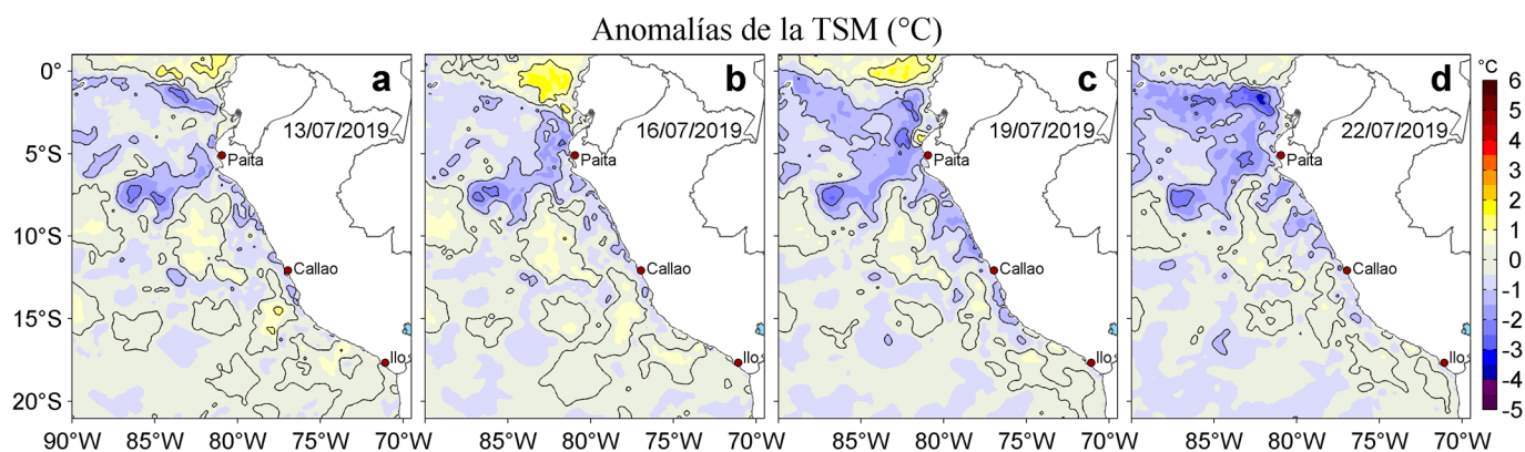
Figura 3. Anomalías de la temperatura superficial del mar (TSM, °C) para los días: a) 13, b) 16, c) 19 y d) 22 de julio de 2019. Las anomalías se calcularon respecto de la climatología para el periodo 2007-2016. Datos: OSTIA-UKMO-L4-GLOB-v2.0 (UK Met Office, 2012; Donlon et al, 2012). Procesamiento: LHF/AFIOF/DGIOCC/IMARPE.
