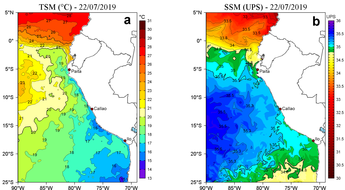
Figura 2. a) Temperatura superficial del mar (TSM, °C) y b) Salinidad superficial del mar (SSM, UPS), para el 22 de julio de 2019. Datos: OSTIA-UKMO-L4-GLOB-v2.0 (UK Met Office, 2012; Donlon et al, 2012) disponible en https://podaac.jpl.nasa.gov/dataset/OSTIA-UKMO-L4-GLOB-v2.0 para (a) y Hybrid Coordinate Ocean Model v. GOFS 3.1 (HYCOM; Halliwell et al., 1998; 2000; Bleck, 2001) para (b). Procesamiento: LHF/AFIOF/DGIOCC/IMARPE.
