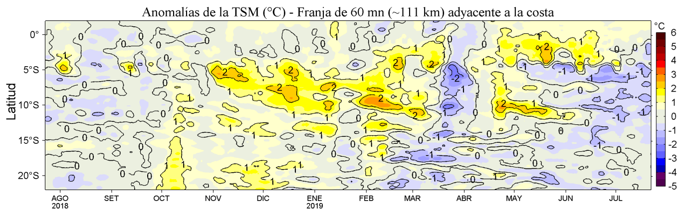
Figura 4. Variación promedio de las anomalías de la temperatura superficial del mar (TSM, °C) para una franja de 60 mn (~111 km) adyacente al litoral peruano para los últimos doce meses al 22 de julio de 2019. Datos: OSTIA-UKMO-L4-GLOB-v2.0 (UK Met. Office, 2012; Donlon et al, 2012) disponible en https://podaac.jpl.nasa.gov/dataset/OSTIA-UKMO-L4-GLOB-v2.0 . Las anomalías se calcularon con respecto al periodo 2007-2016. Procesamiento: LHF/AFIOF/DGIOCC/IMARPE.
