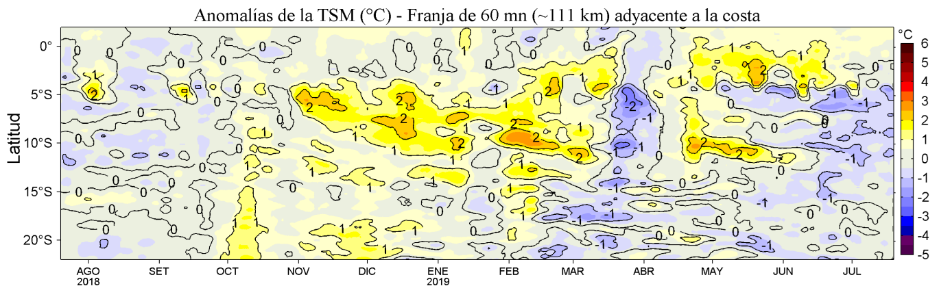
Figura 4. Variación promedio de las anomalías de la temperatura superficial del mar (TSM, °C) para una franja de 60 mn (~111 km) adyacente al litoral peruano para los últimos doce meses al 19 de julio de 2019. Datos: OSTIA-UKMO-L4-GLOB-v2.0 (UK Met. Office, 2012; Donlon et al, 2012) disponible en https://podaac.jpl.nasa.gov/dataset/OSTIA-UKMO-L4-GLOB-v2.0 . Las anomalías se calcularon con respecto al periodo 2007-2016. Procesamiento: LHFM/AFIOF/DGIOCC/IMARPE.
