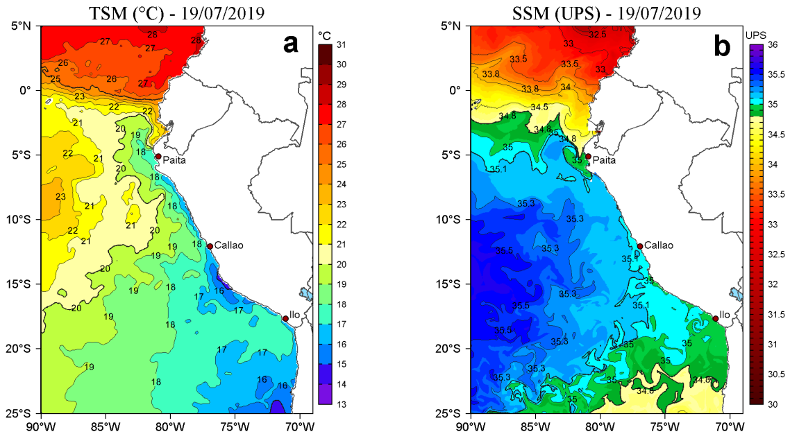
Figura 2. a) Temperatura superficial del mar (TSM, °C) y b) Salinidad superficial del mar (SSM, UPS), para el 19 de julio de 2019. Datos: OSTIA-UKMO-L4-GLOB-v2.0 (UK Met Office, 2012; Donlon et al, 2012) disponible en https://podaac.jpl.nasa.gov/dataset/OSTIA-UKMO-L4-GLOB-v2.0 para (a) y Hybrid Coordinate Ocean Model v. GOFS 3.1 (HYCOM; Halliwell et al., 1998; 2000; Bleck, 2001) para (b). Procesamiento: LHFM/AFIOF/DGIOCC/IMARPE.
