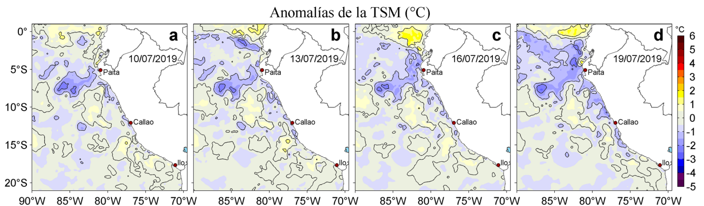
Figura 3. Anomalías de la temperatura superficial del mar (TSM, °C) para los días: a) 10, b) 13, c) 16 y d) 19 de julio de 2019. Las anomalías se calcularon respecto de la climatología para el periodo 2007-2016. Datos: OSTIA-UKMO-L4-GLOB-v2.0 (UK Met Office, 2012; Donlon et al, 2012). Procesamiento: LHFM/AFIOF/DGIOCC/IMARPE.
