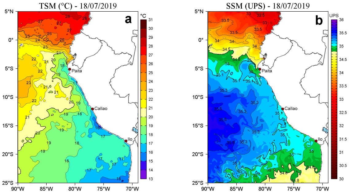
Figura 2. a) Temperatura superficial del mar (TSM, °C) y b) Salinidad superficial del mar (SSM, UPS), para el 18 de julio de 2019. Datos: OSTIA-UKMO-L4-GLOB-v2.0 (UK Met Office, 2012; Donlon et al, 2012) disponible en https://podaac.jpl.nasa.gov/dataset/OSTIA-UKMO-L4-GLOB-v2.0 para (a) y Hybrid Coordinate Ocean Model v. GOF3 3.1 (HYCOM; Halliwell et al., 1998; 2000; Bleck, 2001) para (b). Procesamiento: LHF/M/AFIOF/DGIOCC/IMARPE.
