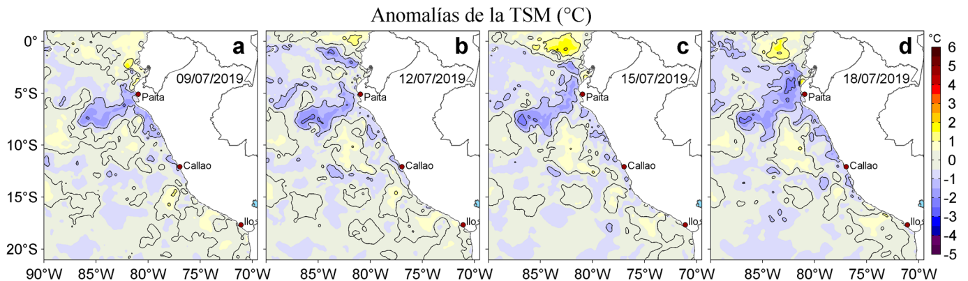
Figura 3. Anomalías de la temperatura superficial del mar (TSM, °C) para los días: a) 09, b) 12, c) 15 y d) 18 de julio de 2019. Las anomalías se calcularon respecto de la climatología para el periodo 2007-2016. Datos: OSTIA-UKMO-L4-GLOB-v2.0 (UK Met Office, 2012; Donlon et al, 2012). Procesamiento: LHF/M/AFIOF/DGIOCC/IMARPE.
