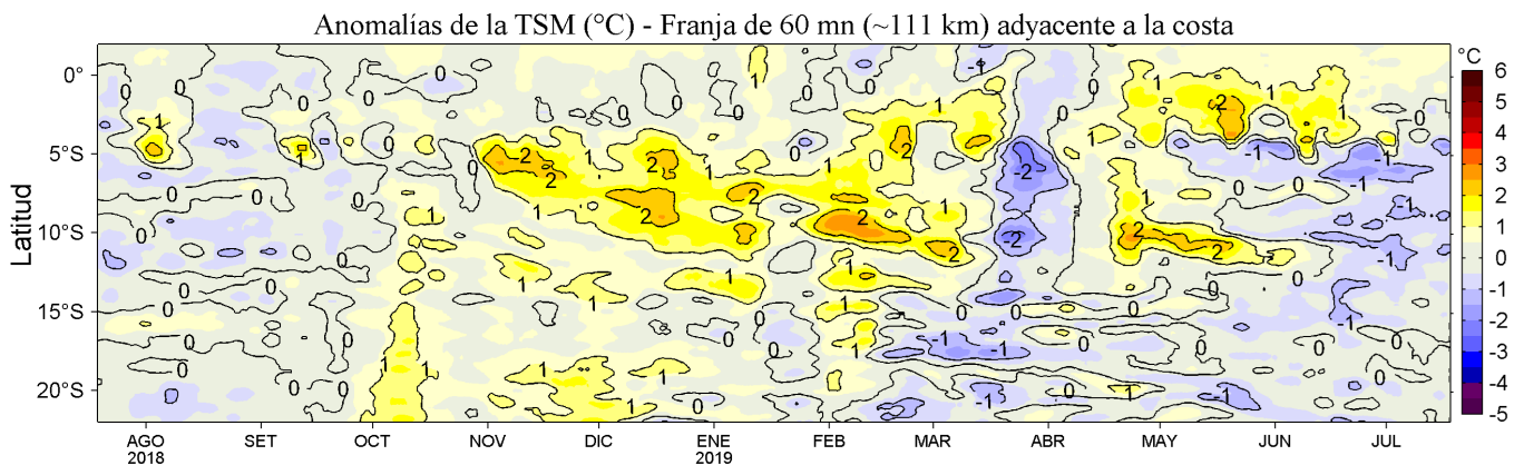
Figura 4. Variación promedio de las anomalías de la temperatura superficial del mar (TSM, °C) para una franja de 60 mn (~111 km) adyacente al litoral peruano para los últimos doce meses al 18 de julio de 2019. Datos: OSTIA-UKMO-L4-GLOB-v2.0 (UK Met. Office, 2012; Donlon et al, 2012) disponible en https://podaac.jpl.nasa.gov/dataset/OSTIA-UKMO-L4-GLOB-v2.0 . Las anomalías se calcularon con respecto al periodo 2007-2016. Procesamiento: LHF/M/AFIOF/DGIOCC/IMARPE.
