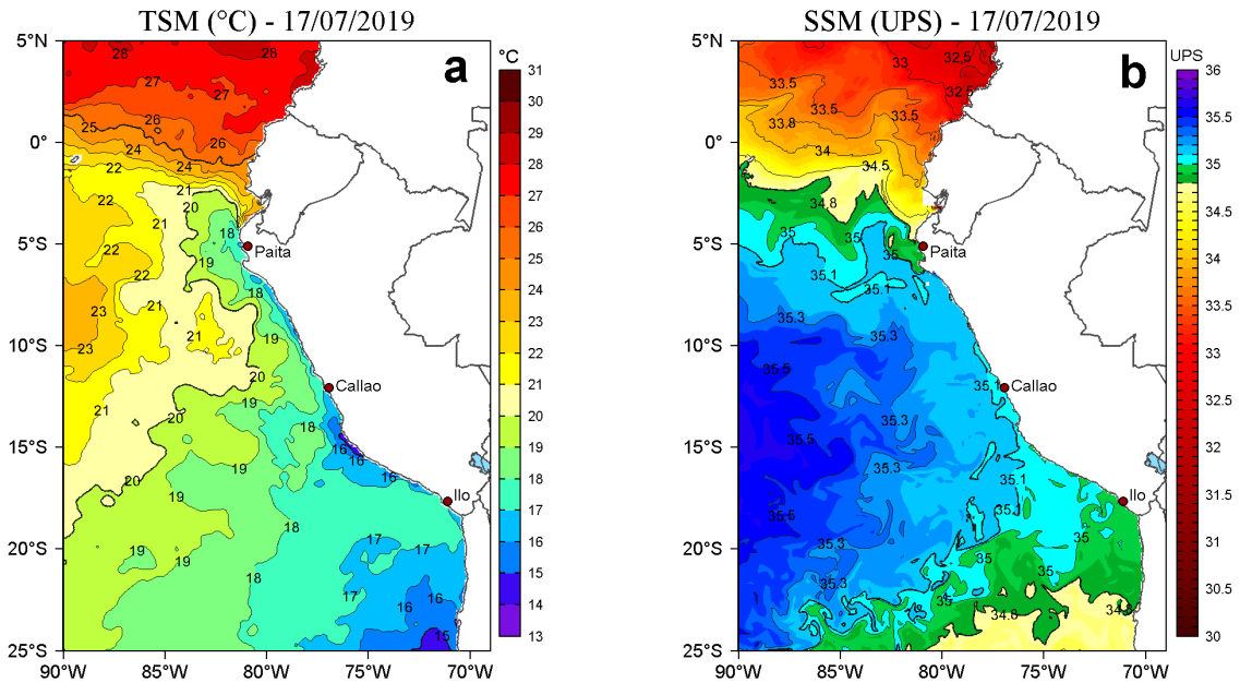
Figura 2. a) Temperatura superficial del mar (TSM, °C) y b) Salinidad superficial del mar (SSM, UPS), para el 17 de julio de 2019. Datos: OSTIA-UKMO-L4-GLOB-v2.0 (UK Met Office, 2012; Donlon et al, 2012) disponible en https://podaac.jpl.nasa.gov/dataset/OSTIA-UKMO-L4-GLOB-v2.0 para (a) y Hybrid Coordinate Ocean Model v. GOFs 3.1 (HYCOM; Halliwell et al., 1998; 2000; Bleck, 2001) para (b). Procesamiento: LHF/AFIOF/DGIOCC/IMARPE.
