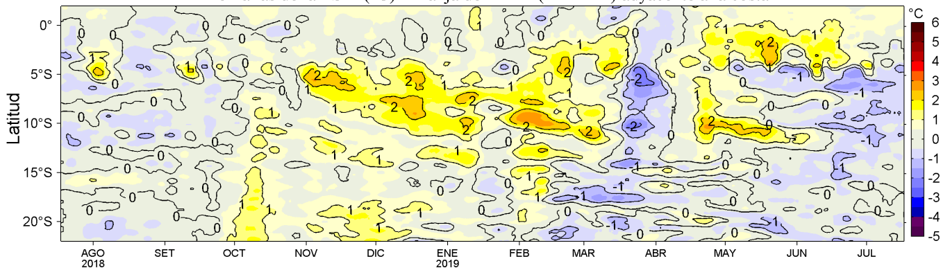
Figura 4. Variación promedio de las anomalías de la temperatura superficial del mar (TSM, °C) para una franja de 60 mn (~111 km) adyacente al litoral peruano para los últimos doce meses al 17 de julio de 2019. Datos: OSTIA-UKMO-L4-GLOB-v2.0 (UK Met. Office, 2012; Donlon et al, 2012) disponible en https://podaac.jpl.nasa.gov/dataset/OSTIA-UKMO-L4-GLOB-v2.0 . Las anomalías se calcularon con respecto al periodo 2007-2016. Procesamiento: LHF/AFIOF/DGIOCC/IMARPE.
