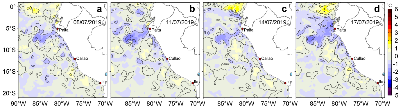
Figura 3. Anomalías de la temperatura superficial del mar (TSM, °C) para los días: a) 08, b) 11, c) 14 y d) 17 de julio de 2019. Las anomalías se calcularon respecto de la climatología para el periodo 2007-2016. Datos: OSTIA-UKMO-L4-GLOB-v2.0 (UK Met Office, 2012; Donlon et al, 2012). Procesamiento: LHF/AFIOF/DGIOCC/IMARPE.
