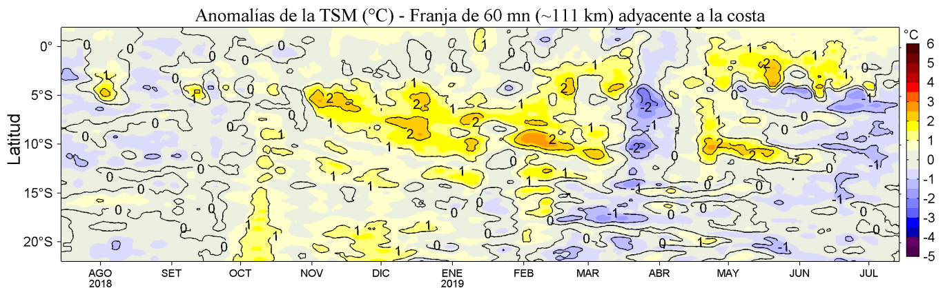
Figura 4. Variación promedio de las anomalías de la temperatura superficial del mar (TSM, °C) para una franja de 60 mn (~111 km) adyacente al litoral peruano para los últimos doce meses al 14 de julio de 2019. Datos: OSTIA-UKMO-L4-GLOB-v2.0 (UK Met. Office, 2012; Donlon et al, 2012) disponible en https://podaac.jpl.nasa.gov/dataset/OSTIA-UKMO-L4-GLOB-v2.0 . Las anomalías se calcularon con respecto al periodo 2007-2016. Procesamiento: LHF/AFIOF/DGIOCC/IMARPE.
