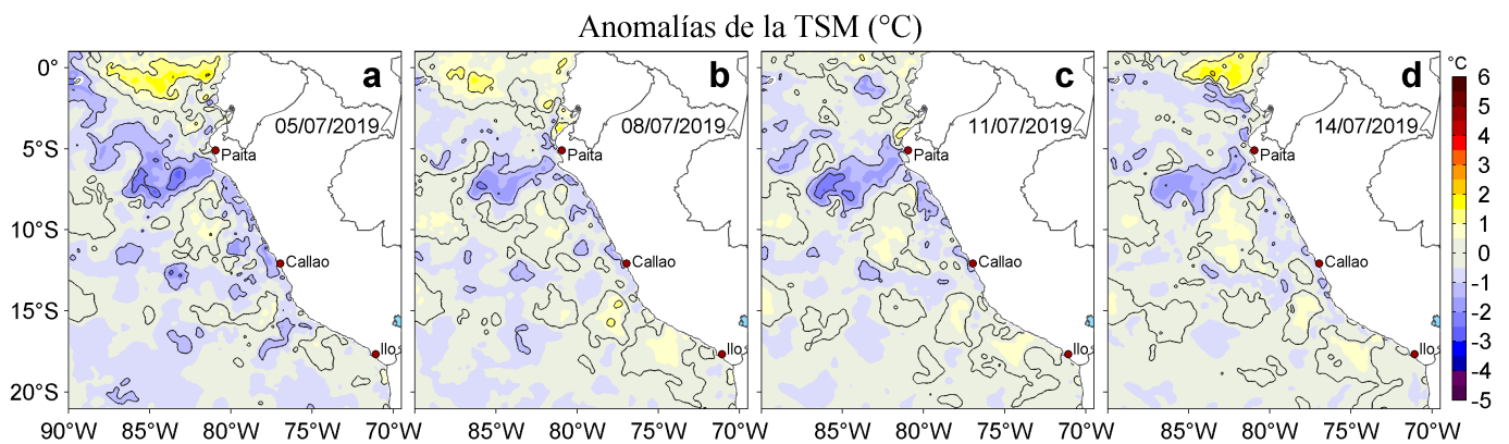
Figura 3. Anomalías de la temperatura superficial del mar (TSM, °C) para los días: a) 05, b) 08, c) 11 y d) 14 de julio de 2019. Las anomalías se calcularon respecto de la climatología para el periodo 2007-2016. Datos: OSTIA-UKMO-L4-GLOB-v2.0 (UK Met Office, 2012; Donlon et al, 2012). Procesamiento: LHF/AFIOF/DGIOCC/IMARPE.
