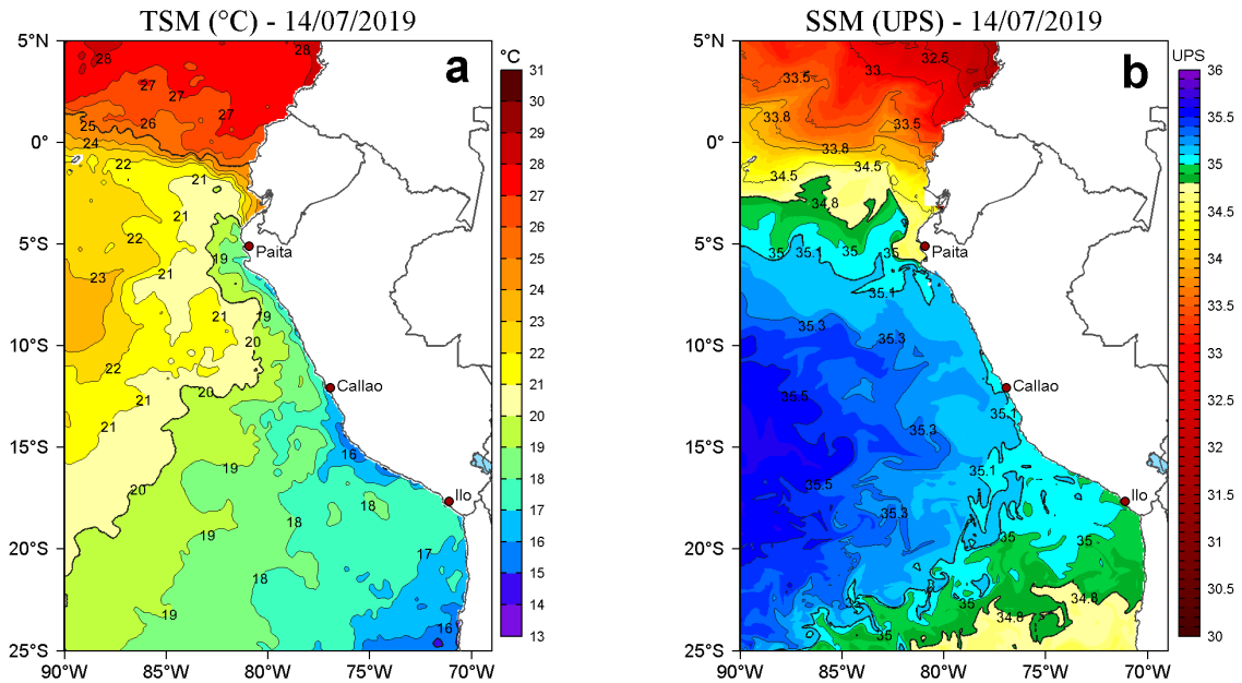
Figura 2. a) Temperatura superficial del mar (TSM, °C) y b) Salinidad superficial del mar (SSM, UPS), para el 14 de julio de 2019. Datos: OSTIA-UKMO-L4-GLOB-v2.0 (UK Met Office, 2012; Donlon et al, 2012) disponible en https://podaac.jpl.nasa.gov/dataset/OSTIA-UKMO-L4-GLOB-v2.0 para (a) y Hybrid Coordinate Ocean Model v. GOF3 3.1 (HYCOM; Halliwell et al., 1998; 2000; Bleck, 2001) para (b). Procesamiento: LHF/AFIOF/DGIOCC/IMARPE.
