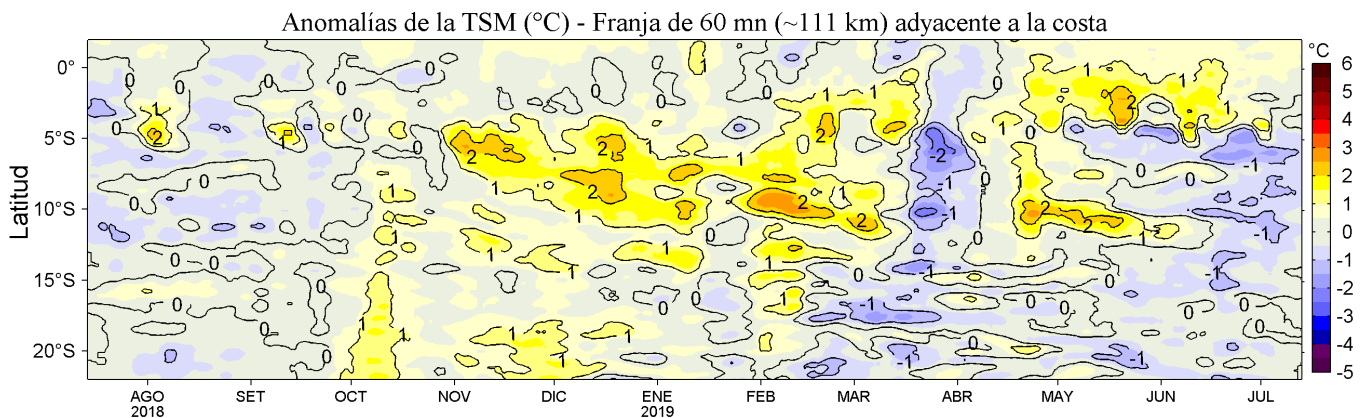
Figura 4. Variación promedio de las anomalías de la temperatura superficial del mar (TSM, °C) para una franja de 60 mn (~111 km) adyacente al litoral peruano para los últimos doce meses al 13 de julio de 2019. Datos: OSTIA-UKMO-L4-GLOB-v2.0 (UK Met. Office, 2012; Donlon et al, 2012) disponible en https://podaac.jpl.nasa.gov/dataset/OSTIA-UKMO-L4-GLOB-v2.0 . Las anomalías se calcularon con respecto al periodo 2007-2016. Procesamiento: LHF/AFIOF/DGIOCC/IMARPE.
