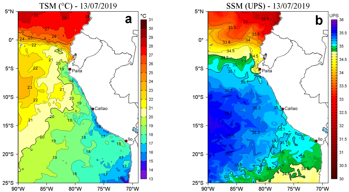
Figura 2. a) Temperatura superficial del mar (TSM, °C) y b) Salinidad superficial del mar (SSM, UPS), para el 13 de julio de 2019. Datos: OSTIA-UKMO-L4-GLOB-v2.0 (UK Met Office, 2012; Donlon et al, 2012) disponible en https://podaac.jpl.nasa.gov/dataset/OSTIA-UKMO-L4-GLOB-v2.0 para (a) y Hybrid Coordinate Ocean Model v. GOFs 3.1 (HYCOM; Halliwell et al., 1998; 2000; Bleck, 2001) para (b). Procesamiento: LHF/AFIOF/DGIOCC/IMARPE.
