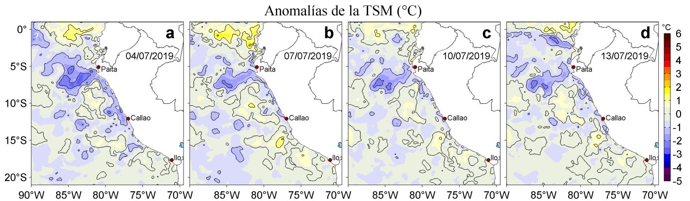
Figura 3. Anomalías de la temperatura superficial del mar (TSM, °C) para los días: a) 04, b) 07, c) 10 y d) 13 de julio de 2019. Las anomalías se calcularon respecto de la climatología para el periodo 2007-2016. Datos: OSTIA-UKMO-L4-GLOB-v2.0 (UK Met Office, 2012; Donlon et al, 2012). Procesamiento: LHF/AFIOF/DGIOCC/IMARPE.
