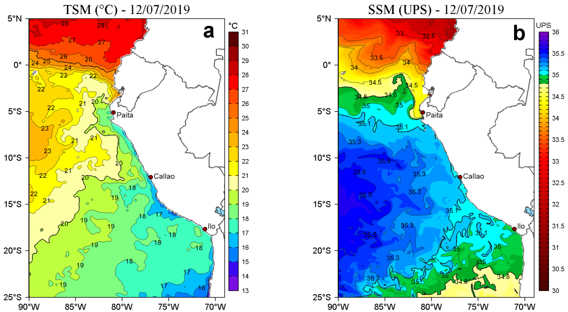
Figura 2. a) Temperatura superficial del mar (TSM, °C) y b) Salinidad superficial del mar (SSM, UPS), para el 12 de julio de 2019. Datos: OSTIA-UKMO-L4-GLOB-v2.0 (UK Met Office, 2012; Donlon et al, 2012) disponible en https://podaac.jpl.nasa.gov/dataset/OSTIA-UKMO-L4-GLOB-v2.0 para (a) y Hybrid Coordinate Ocean Model v. GOF3 3.1 (HYCOM; Halliwell et al., 1998; 2000; Bleck, 2001) para (b). Procesamiento: LHF/AFIOF/DGIOCC/IMARPE.
