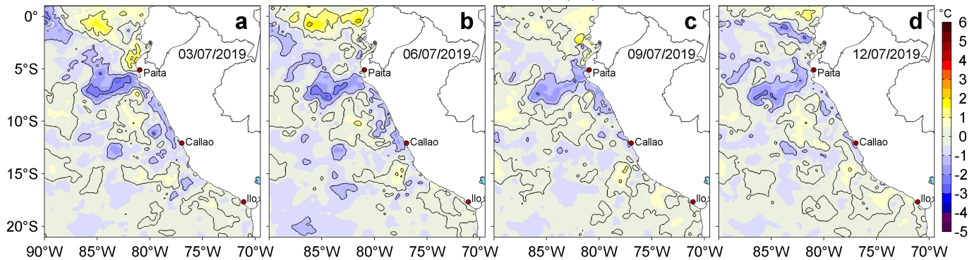
Figura 3. Anomalías de la temperatura superficial del mar (TSM, °C) para los días: a) 03, b) 06, c) 09 y d) 12 de julio de 2019. Las anomalías se calcularon respecto de la climatología para el periodo 2007-2016. Datos: OSTIA-UKMO-L4-GLOB-v2.0 (UK Met Office, 2012; Donlon et al, 2012). Procesamiento: LHF/AFIOF/DGIOCC/IMARPE.
