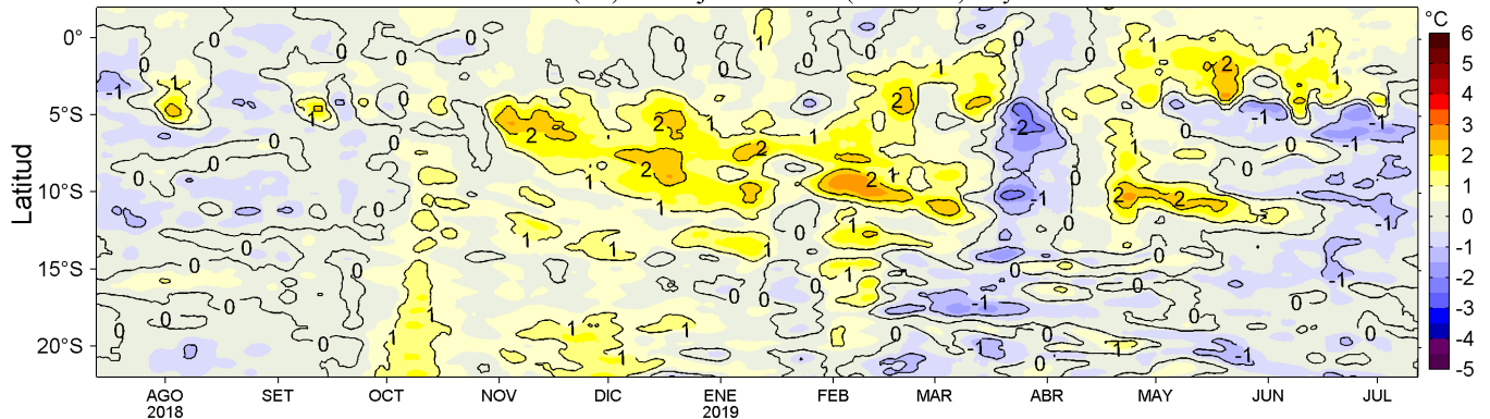
Figura 4. Variación promedio de las anomalías de la temperatura superficial del mar (TSM, °C) para una franja de 60 mn (~111 km) adyacente al litoral peruano para los últimos doce meses al 12 de julio de 2019. Datos: OSTIA-UKMO-L4-GLOB-v2.0 (UK Met. Office, 2012; Donlon et al, 2012) disponible en https://podaac.jpl.nasa.gov/dataset/OSTIA-UKMO-L4-GLOB-v2.0 . Las anomalías se calcularon con respecto al periodo 2007-2016. Procesamiento: LHF/AFIOF/DGIOCC/IMARPE.
