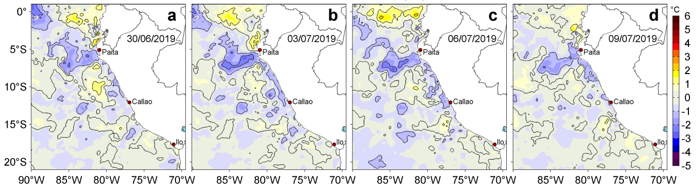
Figura 3. Anomalías de la temperatura superficial del mar (TSM, °C) para los días: a) 30 de junio, b) 03, c) 06 y d) 09 de julio de 2019. Las anomalías se calcularon respecto de la climatología para el periodo 2007-2016. Datos: OSTIA-UKMO-L4-GLOB-v2.0 (UK Met Office, 2012; Donlon et al, 2012). Procesamiento: LHF/AFIOF/DGIOCC/IMARPE.
