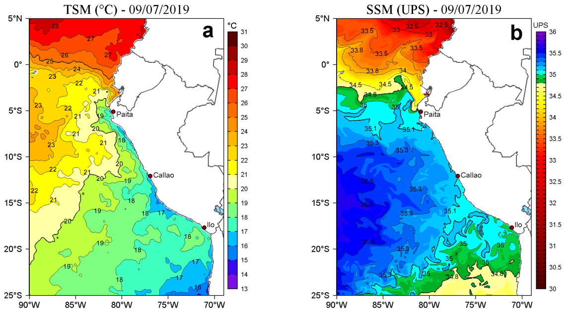
Figura 2. a) Temperatura superficial del mar (TSM, °C) y b) Salinidad superficial del mar (SSM, UPS), para el 09 de julio de 2019. Datos: OSTIA-UKMO-L4-GLOB-v2.0 (UK Met Office, 2012; Donlon et al, 2012) disponible en https://podaac.jpl.nasa.gov/dataset/OSTIA-UKMO-L4-GLOB-v2.0 para (a) y Hybrid Coordinate Ocean Model v. GOF3.1 (HYCOM; Halliwell et al., 1998; 2000; Bleck, 2001) para (b). Procesamiento: LHF/AFIOF/DGIOCC/IMARPE.
