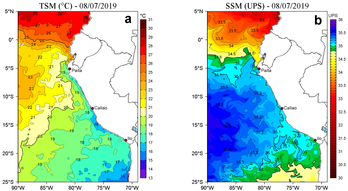
Figura 2. a) Temperatura superficial del mar (TSM, °C) y b) Salinidad superficial del mar (SSM, UPS), para el 08 de julio de 2019. Datos: OSTIA-UKMO-L4-GLOB-v2.0 (UK Met Office, 2012; Donlon et al, 2012) disponible en https://podaac.jpl.nasa.gov/dataset/OSTIA-UKMO-L4-GLOB-v2.0 para (a) y Hybrid Coordinate Ocean Model v. GOF3 3.1 (HYCOM; Halliwell et al., 1998; 2000; Bleck, 2001) para (b). Procesamiento: LHF/AFIOF/DGIOCC/IMARPE.
