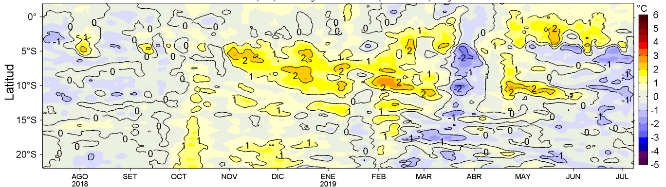
Figura 4. Variación promedio de las anomalías de la temperatura superficial del mar (TSM, °C) para una franja de 60 mn (~111 km) adyacente al litoral peruano para los últimos doce meses al 08 de julio de 2019. Datos: OSTIA-UKMO-L4-GLOB-v2.0 (UK Met. Office, 2012; Donlon et al, 2012) disponible en https://podaac.jpl.nasa.gov/dataset/OSTIA-UKMO-L4-GLOB-v2.0 . Las anomalías se calcularon con respecto al periodo 2007-2016. Procesamiento: LHF/AFIOF/DGIOCC/IMARPE.
