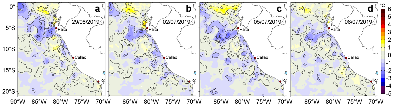
Figura 3. Anomalías de la temperatura superficial del mar (TSM, °C) para los días: a) 29 de junio, b) 02, c) 05 y d) 08 de julio de 2019. Las anomalías se calcularon respecto de la climatología para el periodo 2007-2016. Datos: OSTIA-UKMO-L4-GLOB-v2.0 (UK Met Office, 2012; Donlon et al, 2012). Procesamiento: LHF/AFIOF/DGIOCC/IMARPE.
