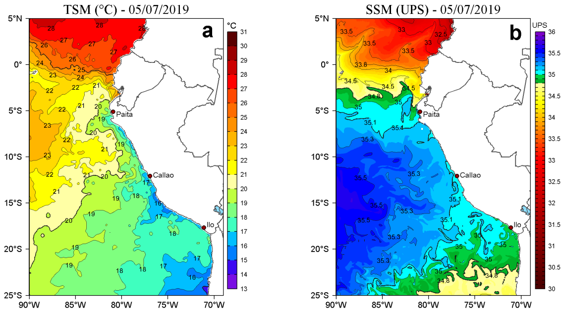
Figura 2. a) Temperatura superficial del mar (TSM, °C) y b) Salinidad superficial del mar (SSM, UPS), para el 05 de julio de 2019. Datos: OSTIA-UKMO-L4-GLOB-v2.0 (UK Met Office, 2012; Donlon et al, 2012) disponible en https://podaac.jpl.nasa.gov/dataset/OSTIA-UKMO-L4-GLOB-v2.0 para (a) y Hybrid Coordinate Ocean Model v. GOF3 3.1 (HYCOM; Halliwell et al., 1998; 2000; Bleck, 2001) para (b). Procesamiento: LHF/AFIOF/DGIOCC/IMARPE.
