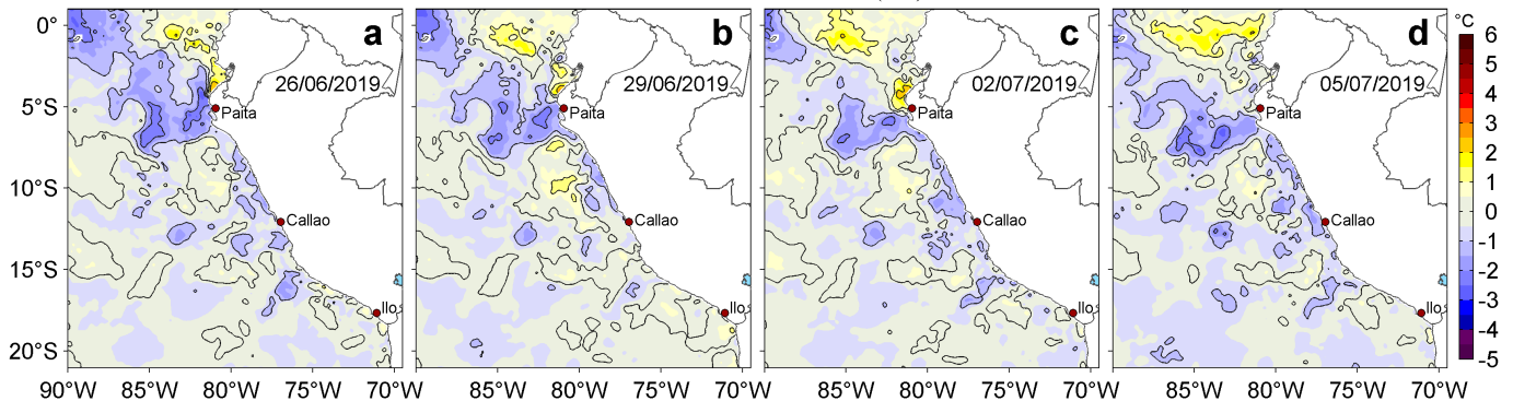
Figura 3. Anomalías de la temperatura superficial del mar (TSM, °C) para los días: a) 26 y b) 29 de junio, c) 02 y d) 05 de julio de 2019. Las anomalías se calcularon respecto de la climatología para el periodo 2007-2016. Datos: OSTIA-UKMO-L4-GLOB-v2.0 (UK Met Office, 2012; Donlon et al, 2012). Procesamiento: LHF/AFIOF/DGIOCC/IMARPE.
