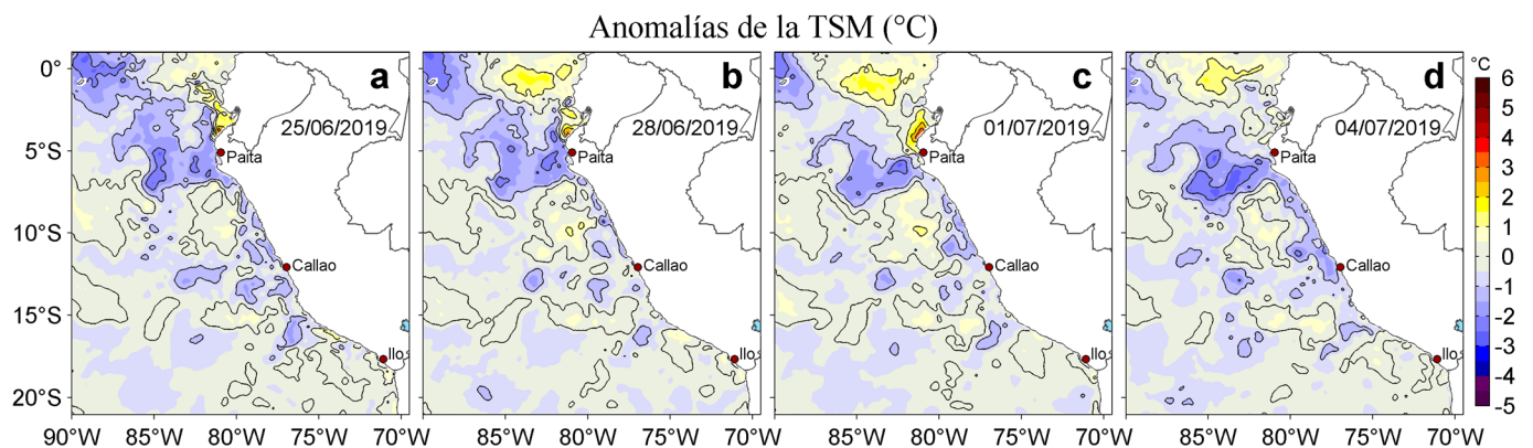
Figura 3. Anomalías de la temperatura superficial del mar (TSM, °C) para los días: a) 25 y b) 28 de junio, c) 01 y d) 04 de julio de 2019. Las anomalías se calcularon respecto de la climatología para el periodo 2007-2016. Datos: OSTIA-UKMO-L4-GLOB-v2.0 (UK Met Office, 2012; Donlon et al, 2012). Procesamiento: LHF/AFIOF/DGIOCC/IMARPE.
