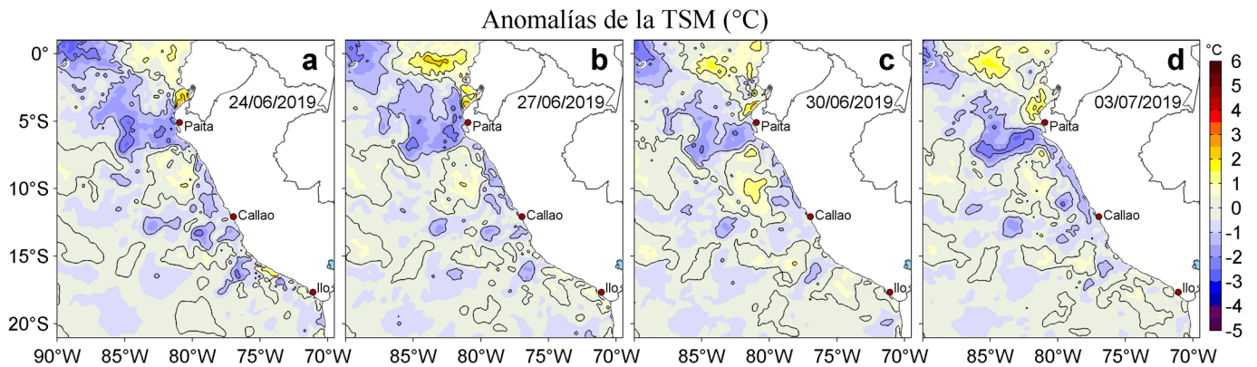
Figura 3. Anomalías de la temperatura superficial del mar (TSM, °C) para los días: a) 24, b) 27 y c) 30 de junio y d) 03 de julio de 2019. Las anomalías se calcularon respecto de la climatología para el periodo 2007-2016. Datos: OSTIA-UKMO-L4-GLOB-v2.0 (UK Met Office, 2012; Donlon et al, 2012). Procesamiento: LHF/AFIOF/DGIOCC/IMARPE.
