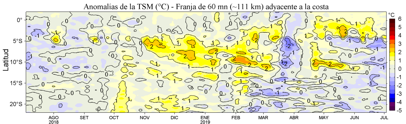
Figura 4. Variación promedio de las anomalías de la temperatura superficial del mar (TSM, °C) para una franja de 60 mn (~111 km) adyacente al litoral peruano para los últimos doce meses al 03 de julio de 2019. Datos: OSTIA-UKMO-L4-GLOB-v2.0 (UK Met. Office, 2012; Donlon et al, 2012) disponible en https://podaac.jpl.nasa.gov/dataset/OSTIA-UKMO-L4-GLOB-v2.0 . Las anomalías se calcularon con respecto al periodo 2007-2016. Procesamiento: LHF/AFIOF/DGIOCC/IMARPE.
