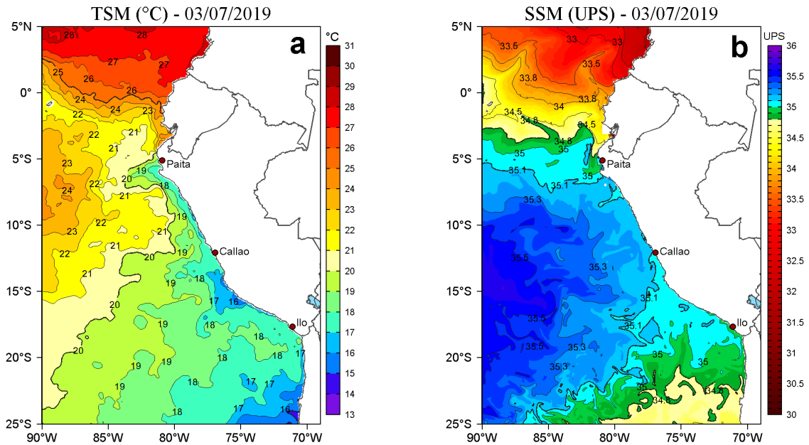
Figura 2. a) Temperatura superficial del mar (TSM, °C) y b) Salinidad superficial del mar (SSM, UPS), para el 03 de julio de 2019. Datos: OSTIA-UKMO-L4-GLOB-v2.0 (UK Met Office, 2012; Donlon et al, 2012) disponible en https://podaac.jpl.nasa.gov/dataset/OSTIA-UKMO-L4-GLOB-v2.0 para (a) y Hybrid Coordinate Ocean Model v. GOFS 3.1 (HYCOM; Halliwell et al., 1998; 2000; Bleck, 2001) para (b). Procesamiento: LHF/AFIOF/DGIOCC/IMARPE.
