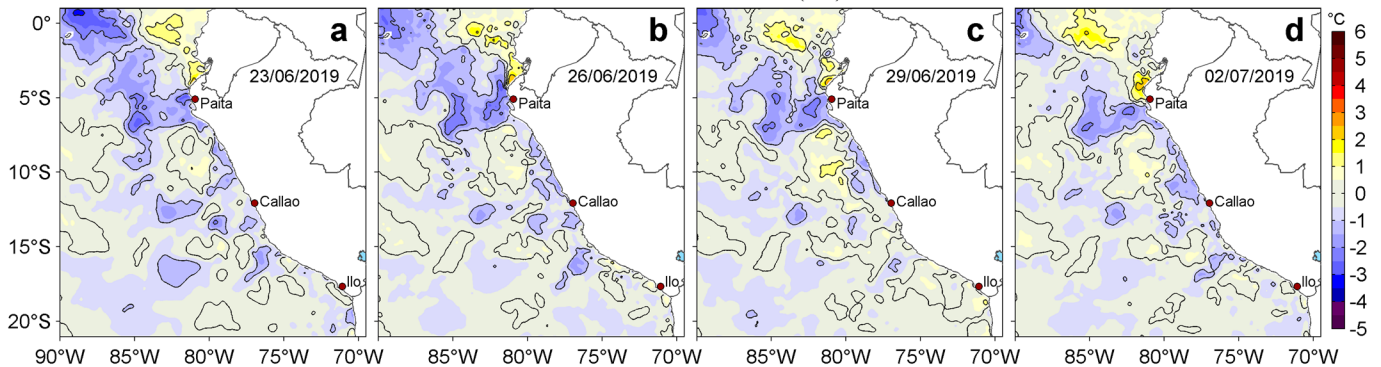
Figura 3. Anomalías de la temperatura superficial del mar (TSM, °C) para los días: a) 23, b) 26 y c) 29 de junio y d) 02 de julio de 2019. Las anomalías se calcularon respecto de la climatología para el periodo 2007-2016. Datos: OSTIA-UKMO-L4-GLOB-v2.0 (UK Met Office, 2012; Donlon et al, 2012). Procesamiento: LHF/AFIOF/DGIOCC/IMARPE.
