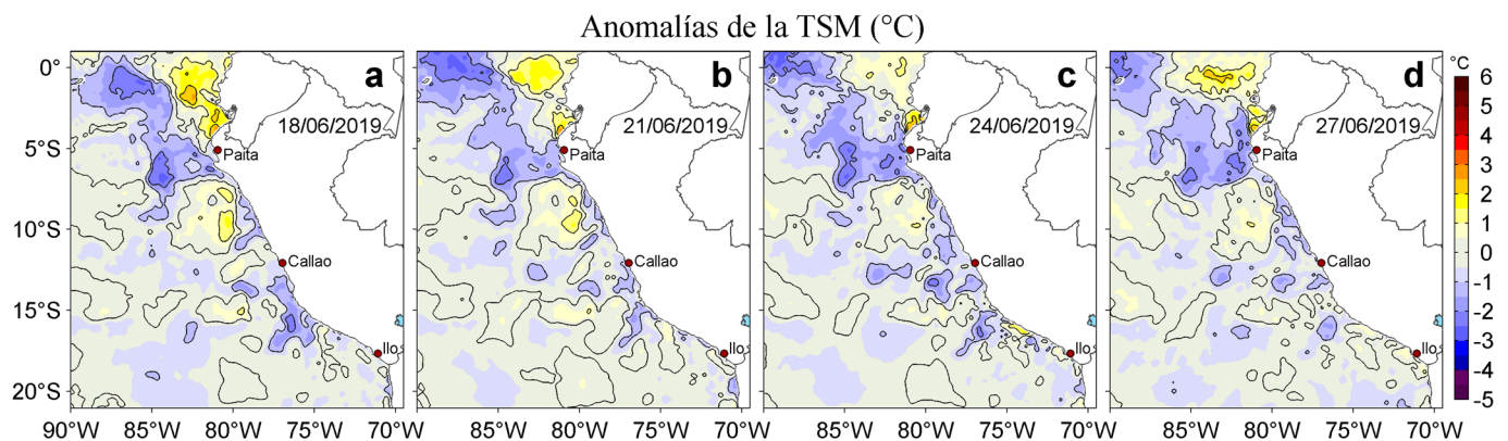
Figura 3. Anomalías de la temperatura superficial del mar (TSM, °C) para los días: a) 18, b) 21, c) 24 y d) 27 de junio de 2019. Las anomalías se calcularon respecto de la climatología para el periodo 2007-2016. Datos: OSTIA-UKMO-L4-GLOB-v2.0 (UK Met Office, 2012; Donlon et al, 2012). Procesamiento: LHF/AFIOF/DGIOCC/IMARPE.
