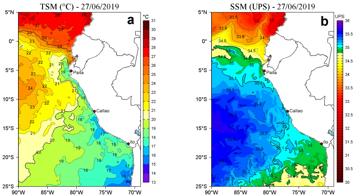
Figura 2. a) Temperatura superficial del mar (TSM, °C) y b) Salinidad superficial del mar (SSM, UPS), para el 27 de junio de 2019. Datos: OSTIA-UKMO-L4-GLOB-v2.0 (UK Met Office, 2012; Donlon et al, 2012) disponible en https://podaac.jpl.nasa.gov/dataset/OSTIA-UKMO-L4-GLOB-v2.0 para (a) y Hybrid Coordinate Ocean Model v. GOFS 3.1 (HYCOM; Halliwell et al., 1998; 2000; Bleck, 2001) para (b). Procesamiento: LHF/AFIOF/DGIOCC/IMARPE.
