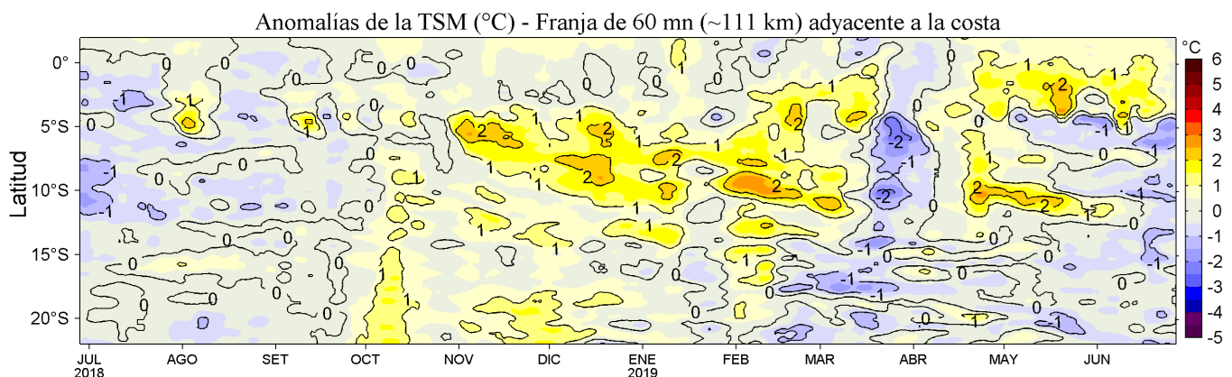
Figura 4. Variación promedio de las anomalías de la temperatura superficial del mar (TSM, °C) para una franja de 60 mn (~111 km) adyacente al litoral peruano para los últimos doce meses al 27 de junio de 2019. Datos: OSTIA-UKMO-L4-GLOB-v2.0 (UK Met. Office, 2012; Donlon et al, 2012) disponible en https://podaac.jpl.nasa.gov/dataset/OSTIA-UKMO-L4-GLOB-v2.0 . Las anomalías se calcularon con respecto al periodo 2007-2016. Procesamiento: LHF/AFIOF/DGIOCC/IMARPE.
