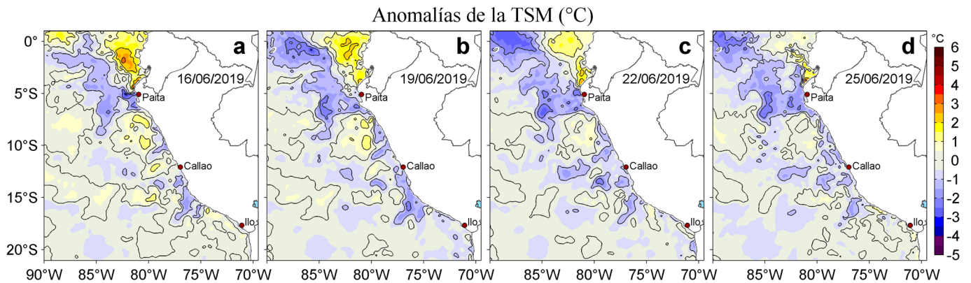
Figura 3. Anomalías de la temperatura superficial del mar (TSM, °C) para los días: a) 16, b) 19, c) 22 y d) 25 de junio de 2019. Las anomalías se calcularon respecto de la climatología para el periodo 2007-2016. Datos: OSTIA-UKMO-L4-GLOB-v2.0 (UK Met Office, 2012; Donlon et al, 2012). Procesamiento: LHFM/AFIOF/DGIOCC/IMARPE.
