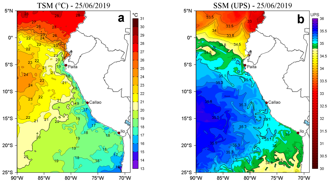
Figura 2. a) Temperatura superficial del mar (TSM, °C) y b) Salinidad superficial del mar (SSM, UPS), para el 25 de junio de 2019. Datos: OSTIA-UKMO-L4-GLOB-v2.0 (UK Met Office, 2012; Donlon et al, 2012) disponible en https://podaac.jpl.nasa.gov/dataset/OSTIA-UKMO-L4-GLOB-v2.0 para (a) y Hybrid Coordinate Ocean Model v. GOFS 3.1 (HYCOM; Halliwell et al., 1998; 2000; Bleck, 2001) para (b). Procesamiento: LHFM/AFIOF/DGIOCC/IMARPE.
