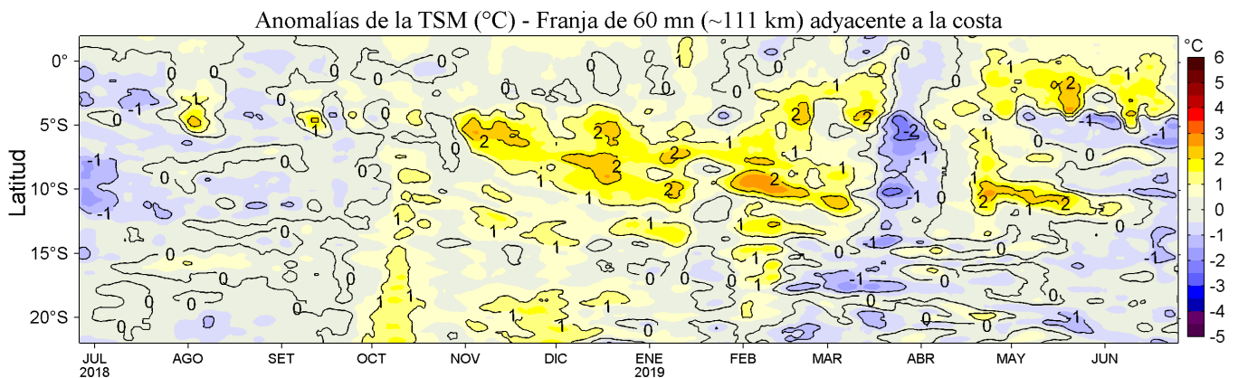
Figura 4. Variación promedio de las anomalías de la temperatura superficial del mar (TSM, °C) para una franja de 60 mn (~111 km) adyacente al litoral peruano para los últimos doce meses al 25 de junio de 2019. Datos: OSTIA-UKMO-L4-GLOB-v2.0 (UK Met. Office, 2012; Donlon et al, 2012) disponible en https://podaac.jpl.nasa.gov/dataset/OSTIA-UKMO-L4-GLOB-v2.0 . Las anomalías se calcularon con respecto al periodo 2007-2016. Procesamiento: LHFM/AFIOF/DGIOCC/IMARPE.
