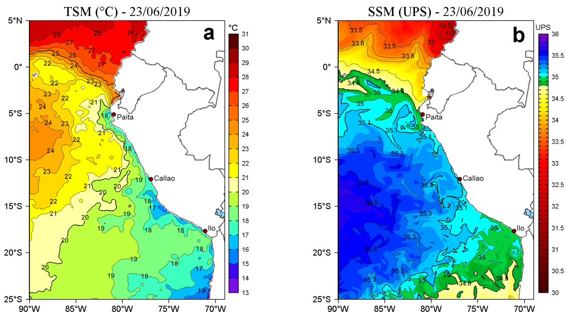
Figura 2. a) Temperatura superficial del mar (TSM, °C) y b) Salinidad superficial del mar (SSM, UPS), para el 23 de junio de 2019. Datos: OSTIA-UKMO-L4-GLOB-v2.0 (UK Met Office, 2012; Donlon et al, 2012) disponible en https://podaac.jpl.nasa.gov/dataset/OSTIA-UKMO-L4-GLOB-v2.0 para (a) y Hybrid Coordinate Ocean Model v. GOFS 3.1 (HYCOM; Halliwell et al., 1998; 2000; Bleck, 2001) para (b). Procesamiento: LHFM/AFIOF/DGIOCC/IMARPE.
