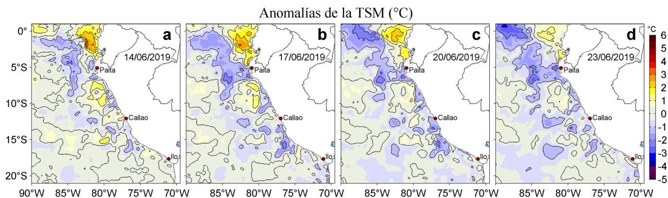
Figura 3. Anomalías de la temperatura superficial del mar (TSM, °C) para los días: a) 14, b) 17, c) 20 y d) 23 de junio de 2019. Las anomalías se calcularon respecto de la climatología para el periodo 2007-2016. Datos: OSTIA-UKMO-L4-GLOB-v2.0 (UK Met Office, 2012; Donlon et al, 2012). Procesamiento: LHFM/AFIOF/DGIOCC/IMARPE.
