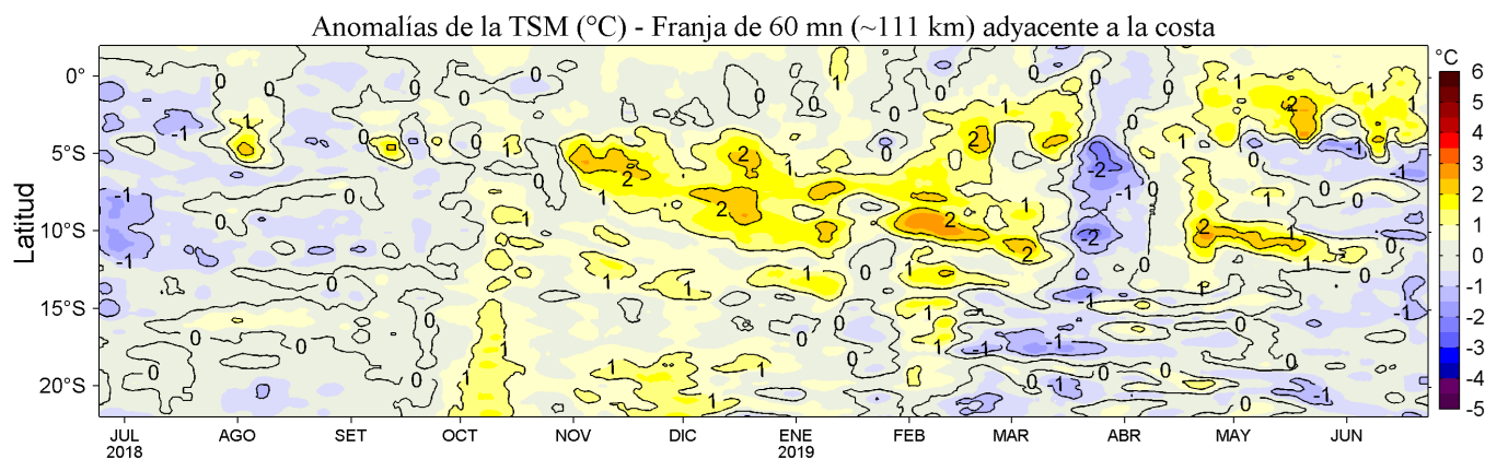
Figura 4. Variación promedio de las anomalías de la temperatura superficial del mar (TSM, °C) para una franja de 60 mn (~111 km) adyacente al litoral peruano para los últimos doce meses al 23 de junio de 2019. Datos: OSTIA-UKMO-L4-GLOB-v2.0 (UK Met. Office, 2012; Donlon et al, 2012) disponible en https://podaac.jpl.nasa.gov/dataset/OSTIA-UKMO-L4-GLOB-v2.0 . Las anomalías se calcularon con respecto al periodo 2007-2016. Procesamiento: LHFM/AFIOF/DGIOCC/IMARPE.
