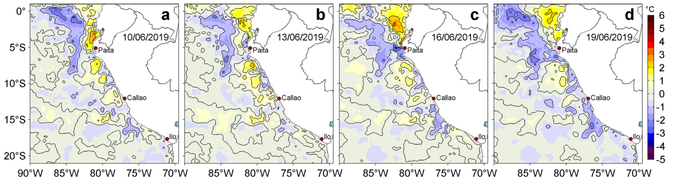
Figura 3. Anomalías de la temperatura superficial del mar (TSM, °C) para los días: a) 10, b) 13, c) 16 y d) 19 de junio de 2019. Las anomalías se calcularon respecto de la climatología para el periodo 2007-2016. Datos: OSTIA-UKMO-L4-GLOB-v2.0 (UK Met Office, 2012; Donlon et al, 2012). Procesamiento: LHFM/AFIOF/DGIOCC/IMARPE.
