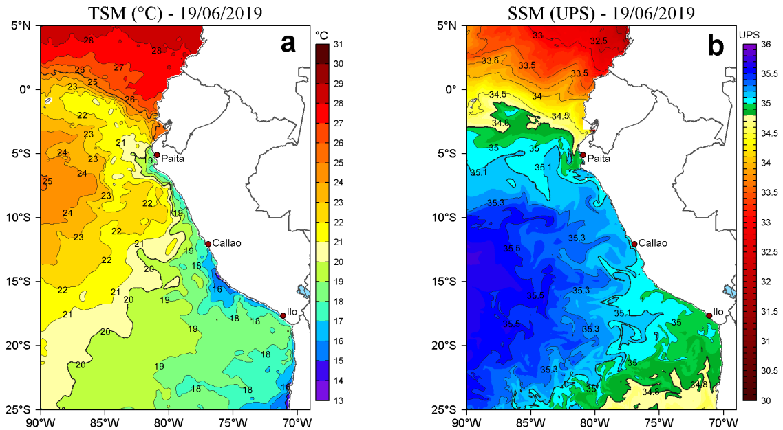
Figura 2. a) Temperatura superficial del mar (TSM, °C) y b) Salinidad superficial del mar (SSM, UPS), para el 19 de junio de 2019. Datos: OSTIA-UKMO-L4-GLOB-v2.0 (UK Met Office, 2012; Donlon et al, 2012) disponible en https://podaac.jpl.nasa.gov/dataset/OSTIA-UKMO-L4-GLOB-v2.0 para (a) y Hybrid Coordinate Ocean Model v. GOF3 3.1 (HYCOM; Halliwell et al., 1998; 2000; Bleck, 2001) para (b). Procesamiento: LHFM/AFIOF/DGIOCC/IMARPE.
