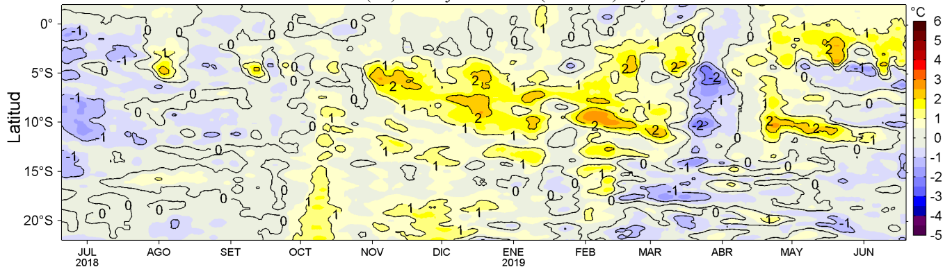
Figura 4. Variación promedio de las anomalías de la temperatura superficial del mar (TSM, °C) para una franja de 60 mn (~111 km) adyacente al litoral peruano para los últimos doce meses al 19 de junio de 2019. Datos: OSTIA-UKMO-L4-GLOB-v2.0 (UK Met. Office, 2012; Donlon et al, 2012) disponible en https://podaac.jpl.nasa.gov/dataset/OSTIA-UKMO-L4-GLOB-v2.0 . Las anomalías se calcularon con respecto al periodo 2007-2016. Procesamiento: LHFM/AFIOF/DGIOCC/IMARPE.
