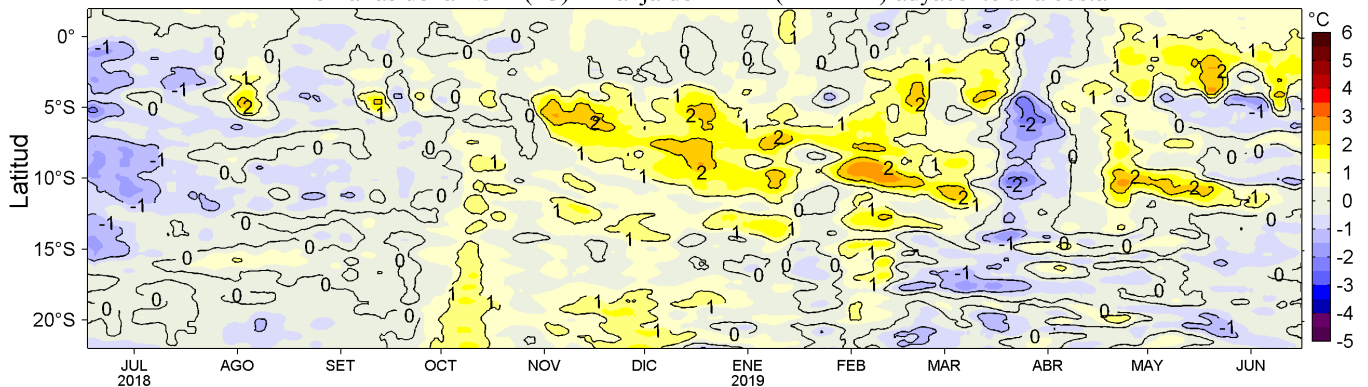
Figura 4. Variación promedio de las anomalías de la temperatura superficial del mar (TSM, °C) para una franja de 60 mn (~111 km) adyacente al litoral peruano para los últimos doce meses al 16 de junio de 2019. Datos: OSTIA-UKMO-L4-GLOB-v2.0 (UK Met. Office, 2012; Donlon et al, 2012) disponible en https://podaac.jpl.nasa.gov/dataset/OSTIA-UKMO-L4-GLOB-v2.0 . Las anomalías se calcularon con respecto al periodo 2007-2016. Procesamiento: LHF/AFIOF/DGIOCC/IMARPE.
