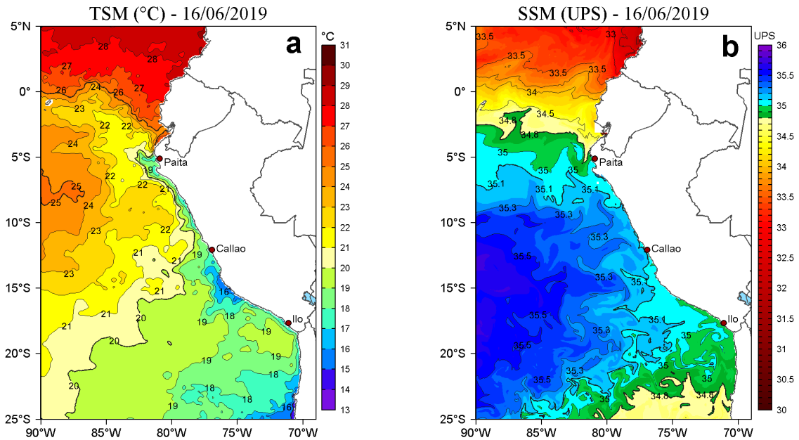
Figura 2. a) Temperatura superficial del mar (TSM, °C) y b) Salinidad superficial del mar (SSM, UPS), para el 16 de junio de 2019. Datos: OSTIA-UKMO-L4-GLOB-v2.0 (UK Met Office, 2012; Donlon et al, 2012) disponible en https://podaac.jpl.nasa.gov/dataset/OSTIA-UKMO-L4-GLOB-v2.0 para (a) y Hybrid Coordinate Ocean Model v. GOF3 3.1 (HYCOM; Halliwell et al., 1998; 2000; Bleck, 2001) para (b). Procesamiento: LHF/AFIOF/DGIOCC/IMARPE.
