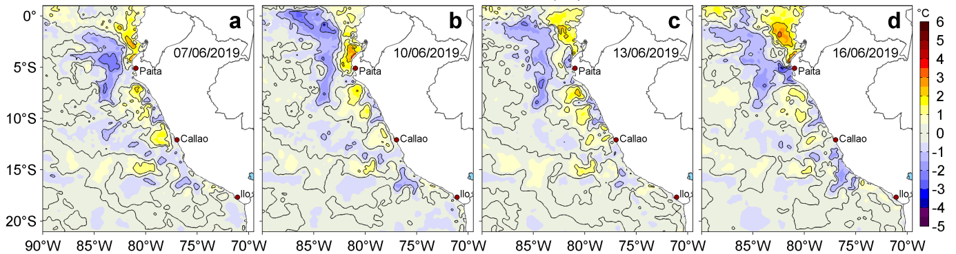
Figura 3. Anomalías de la temperatura superficial del mar (TSM, °C) para los días: a) 07, b) 10, c) 13 y d) 16 de junio de 2019. Las anomalías se calcularon respecto de la climatología para el periodo 2007-2016. Datos: OSTIA-UKMO-L4-GLOB-v2.0 (UK Met Office, 2012; Donlon et al, 2012). Procesamiento: LHF/AFIOF/DGIOCC/IMARPE.
