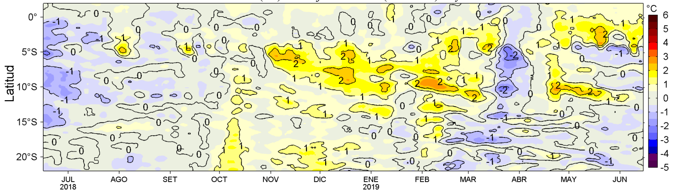
Figura 4. Variación promedio de las anomalías de la temperatura superficial del mar (TSM, °C) para una franja de 60 mn (~111 km) adyacente al litoral peruano para los últimos doce meses al 15 de junio de 2019. Datos: OSTIA-UKMO-L4-GLOB-v2.0 (UK Met. Office, 2012; Donlon et al, 2012) disponible en https://podaac.jpl.nasa.gov/dataset/OSTIA-UKMO-L4-GLOB-v2.0 . Las anomalías se calcularon con respecto al periodo 2007-2016. Procesamiento: LHF/AFIOF/DGIOCC/IMARPE.
