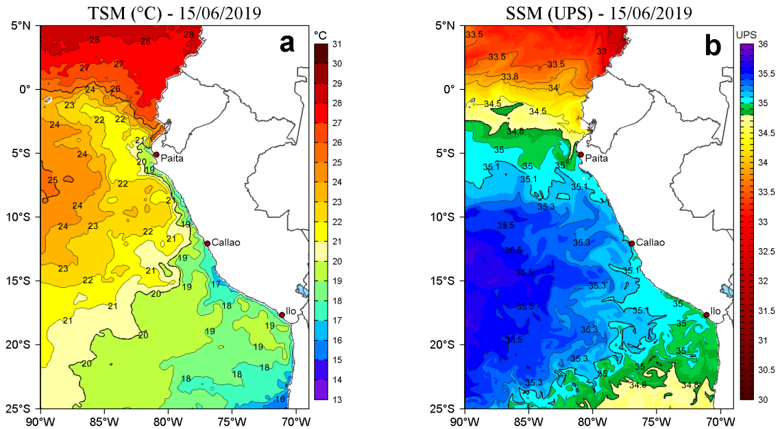
Figura 2. a) Temperatura superficial del mar (TSM, °C) y b) Salinidad superficial del mar (SSM, UPS), para el 15 de junio de 2019. Datos: OSTIA-UKMO-L4-GLOB-v2.0 (UK Met Office, 2012; Donlon et al, 2012) disponible en https://podaac.jpl.nasa.gov/dataset/OSTIA-UKMO-L4-GLOB-v2.0 para (a) y Hybrid Coordinate Ocean Model v. GOF5 3.1 (HYCOM; Halliwell et al., 1998; 2000; Bleck, 2001) para (b). Procesamiento: LHF/AFIOF/DGIOCC/IMARPE.
