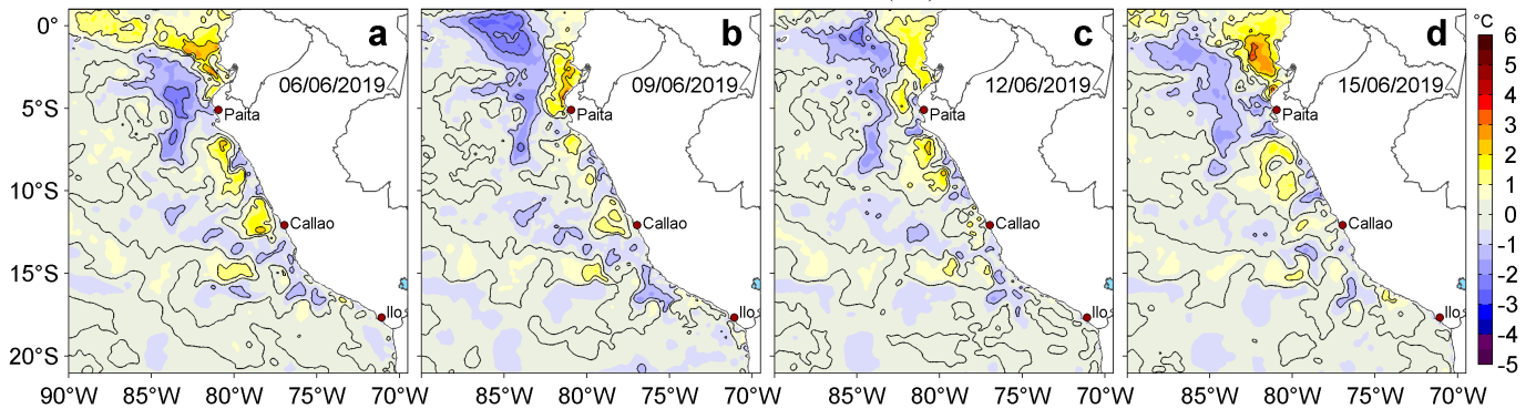
Figura 3. Anomalías de la temperatura superficial del mar (TSM, °C) para los días: a) 06, b) 09, c) 12 y d) 15 de junio de 2019. Las anomalías se calcularon respecto de la climatología para el periodo 2007-2016. Datos: OSTIA-UKMO-L4-GLOB-v2.0 (UK Met Office, 2012; Donlon et al, 2012). Procesamiento: LHF/AFIOF/DGIOCC/IMARPE.
