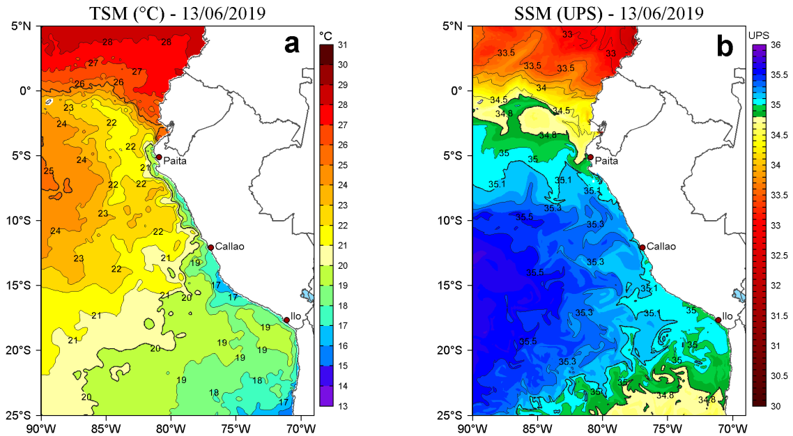
Figura 2. a) Temperatura superficial del mar (TSM, °C) y b) Salinidad superficial del mar (SSM, UPS), para el 13 de junio de 2019. Datos: OSTIA-UKMO-L4-GLOB-v2.0 (UK Met Office, 2012; Donlon et al, 2012) disponible en https://podaac.jpl.nasa.gov/dataset/OSTIA-UKMO-L4-GLOB-v2.0 para (a) y Hybrid Coordinate Ocean Model v. GOFS 3.1 (HYCOM; Halliwell et al., 1998; 2000; Bleck, 2001) para (b). Procesamiento: LHF/M/AFIOF/DGIOCC/IMARPE.
