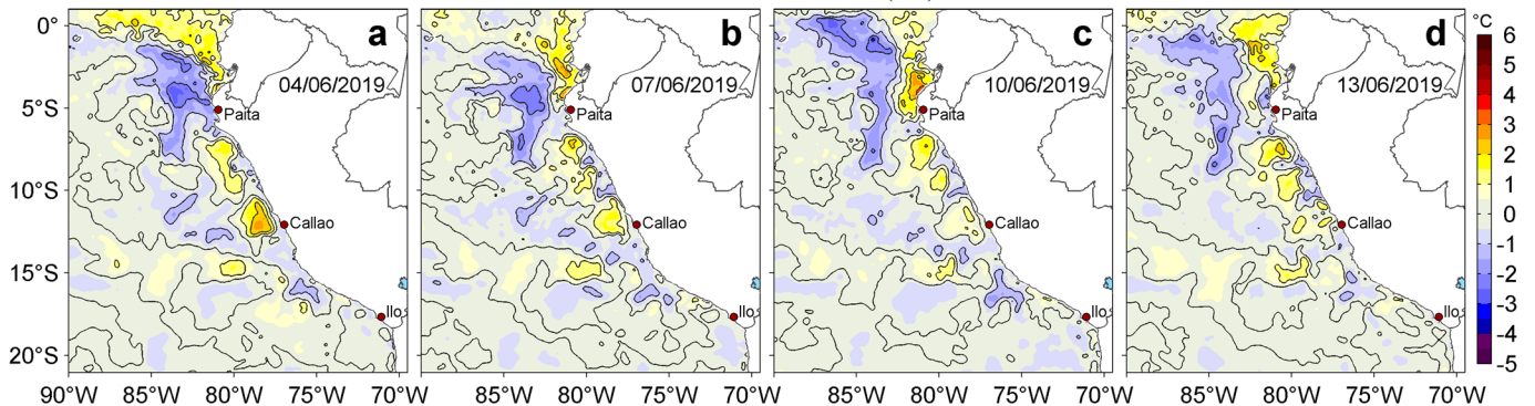
Figura 3. Anomalías de la temperatura superficial del mar (TSM, °C) para los días: a) 04, b) 07, c) 10 y d) 13 de junio de 2019. Las anomalías se calcularon respecto de la climatología para el periodo 2007-2016. Datos: OSTIA-UKMO-L4-GLOB-v2.0 (UK Met Office, 2012; Donlon et al, 2012). Procesamiento: LHF/M/AFIOF/DGIOCC/IMARPE.
