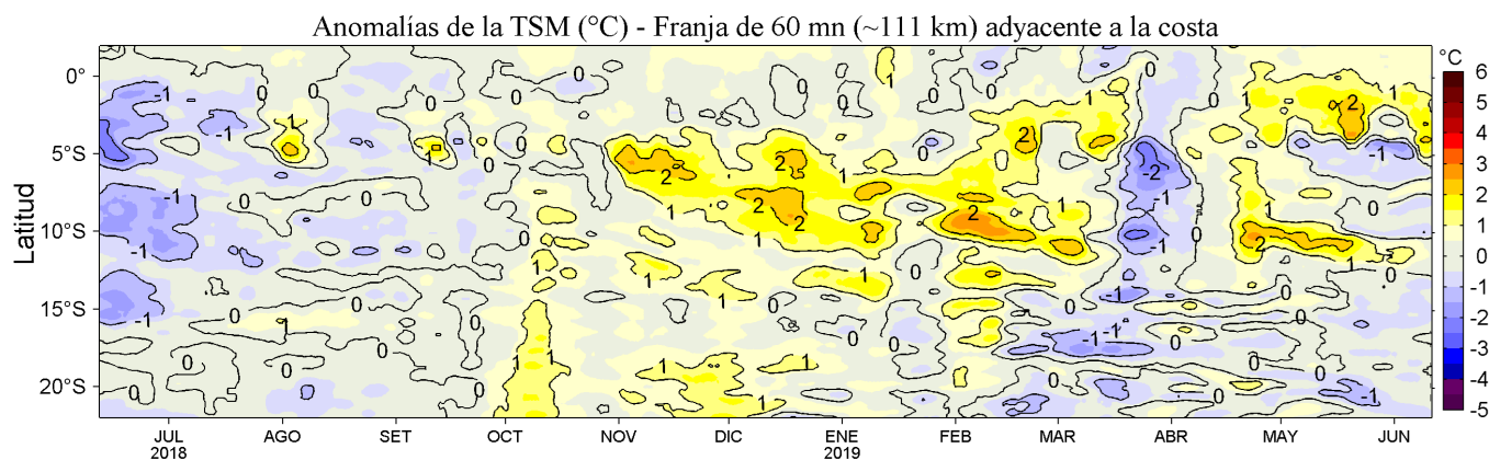
Figura 4. Variación promedio de las anomalías de la temperatura superficial del mar (TSM, °C) para una franja de 60 mn (~111 km) adyacente al litoral peruano para los últimos doce meses al 11 de junio de 2019. Datos: OSTIA-UKMO-L4-GLOB-v2.0 (UK Met. Office, 2012; Donlon et al, 2012) disponible en https://podaac.jpl.nasa.gov/dataset/OSTIA-UKMO-L4-GLOB-v2.0 . Las anomalías se calcularon con respecto al periodo 2007-2016. Procesamiento: LHF/AFIOF/DGIOCC/IMARPE.
