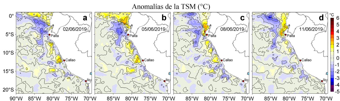
Figura 3. Anomalías de la temperatura superficial del mar (TSM, °C) para los días: a) 02, b) 05, c) 08 y d) 11 de junio de 2019. Las anomalías se calcularon respecto de la climatología para el periodo 2007-2016. Datos: OSTIA-UKMO-L4-GLOB-v2.0 (UK Met Office, 2012; Donlon et al, 2012). Procesamiento: LHF/AFIOF/DGIOCC/IMARPE.
