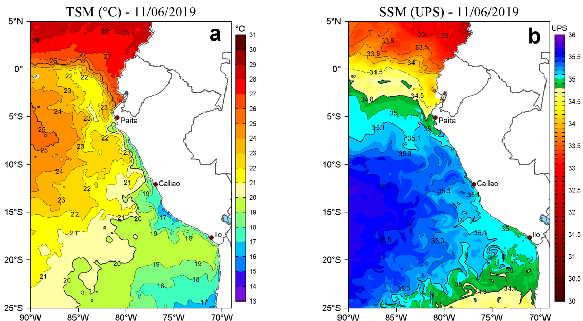
Figura 2. a) Temperatura superficial del mar (TSM, °C) y b) Salinidad superficial del mar (SSM, UPS), para el 11 de junio de 2019. Datos: OSTIA-UKMO-L4-GLOB-v2.0 (UK Met Office, 2012; Donlon et al, 2012) disponible en https://podaac.jpl.nasa.gov/dataset/OSTIA-UKMO-L4-GLOB-v2.0 para (a) y Hybrid Coordinate Ocean Model v. GOFS 3.1 (HYCOM; Halliwell et al., 1998; 2000; Bleck, 2001) para (b). Procesamiento: LHF/AFIOF/DGIOCC/IMARPE.
