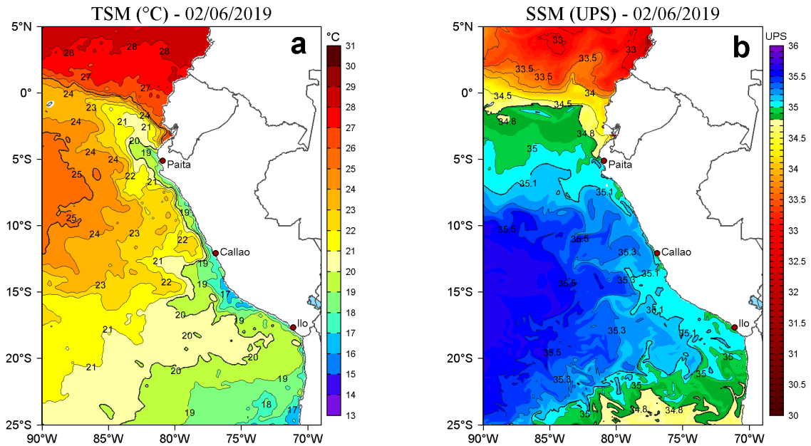
Figura 2. a) Temperatura superficial del mar (TSM, °C) y b) Salinidad superficial del mar (SSM, UPS), para el 02 de junio de 2019. Datos: OSTIA-UKMO-L4-GLOB-v2.0 (UK Met Office, 2012; Donlon et al, 2012) disponible en https://podaac.jpl.nasa.gov/dataset/OSTIA-UKMO-L4-GLOB-v2.0 para (a) y Hybrid Coordinate Ocean Model v. GOF5 3.1 (HYCOM; Halliwell et al., 1998; 2000; Bleck, 2001) para (b). Procesamiento: LHF/AFIOF/DGIOCC/IMARPE.
