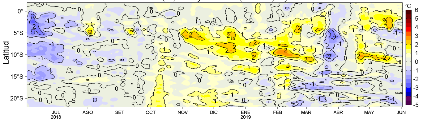
Figura 4. Variación promedio de las anomalías de la temperatura superficial del mar (TSM, °C) para una franja de 60 mn (~111 km) adyacente al litoral peruano para los últimos doce meses al 02 de junio de 2019. Datos: OSTIA-UKMO-L4-GLOB-v2.0 (UK Met. Office, 2012; Donlon et al, 2012) disponible en https://podaac.jpl.nasa.gov/dataset/OSTIA-UKMO-L4-GLOB-v2.0 . Las anomalías se calcularon con respecto al periodo 2007-2016. Procesamiento: LHF/AFIOF/DGIOCC/IMARPE.
