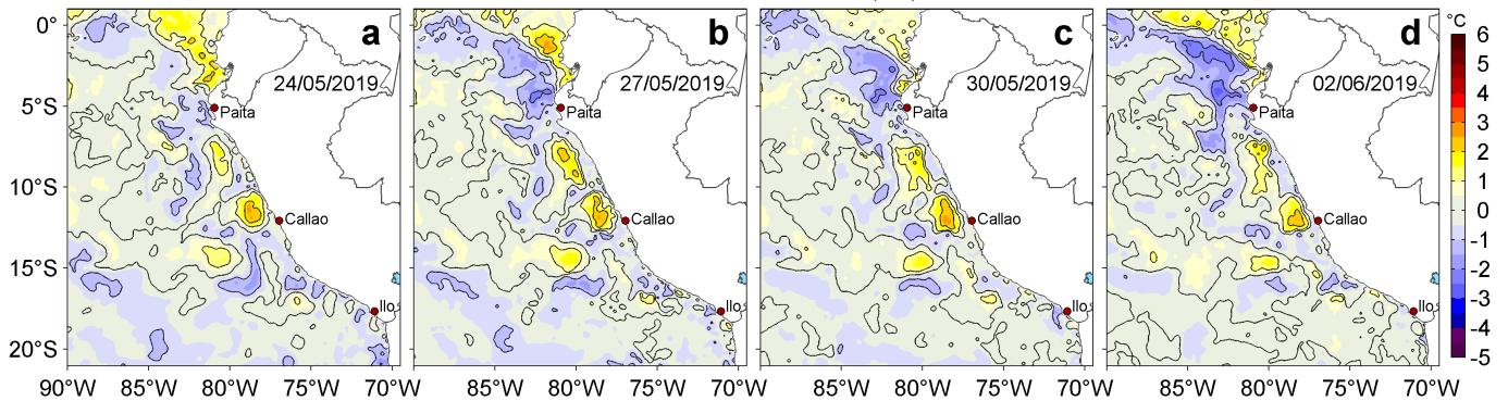
Figura 3. Anomalías de la temperatura superficial del mar (TSM, °C) para los días: a) 24, b) 27 y c) 30 de mayo y d) 02 de junio de 2019. Las anomalías se calcularon respecto de la climatología para el periodo 2007-2016. Datos: OSTIA-UKMO-L4-GLOB-v2.0 (UK Met Office, 2012; Donlon et al, 2012). Procesamiento: LHF/AFIOF/DGIOCC/IMARPE.
