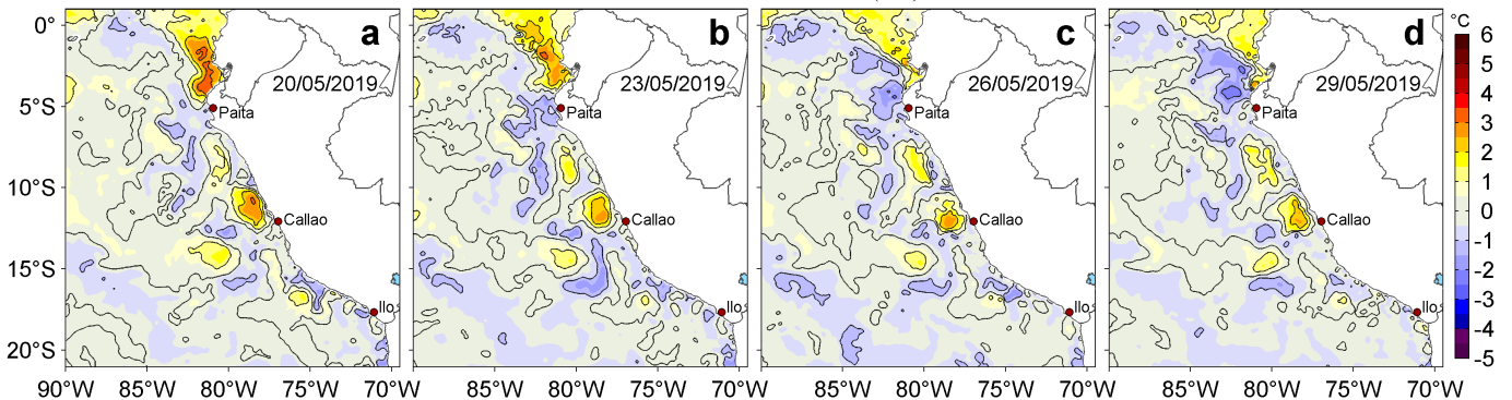
Figura 3. Anomalías de la temperatura superficial del mar (TSM, °C) para los días: a) 20, b) 23, c) 26 y d) 29 de mayo de 2019. Las anomalías se calcularon respecto de la climatología para el periodo 2007-2016. Datos: OSTIA-UKMO-L4-GLOB-v2.0 (UK Met Office, 2012; Donlon et al, 2012). Procesamiento: LHF/AFIOF/DGIOCC/IMARPE.
