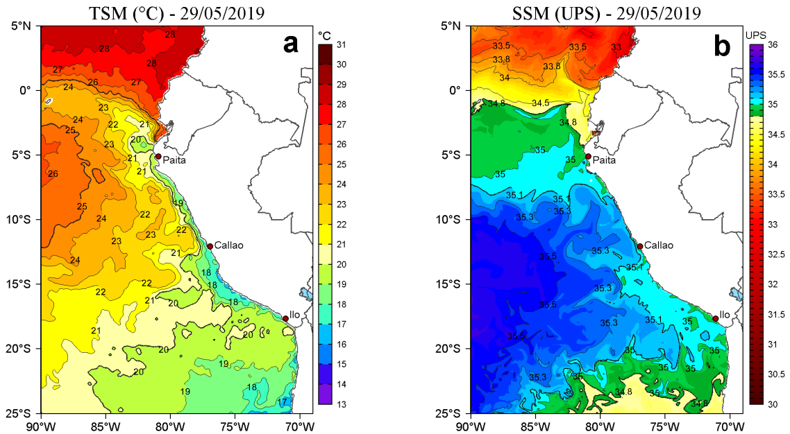
Figura 2. a) Temperatura superficial del mar (TSM, °C) y b) Salinidad superficial del mar (SSM, UPS), para el 29 de mayo de 2019. Datos: OSTIA-UKMO-L4-GLOB-v2.0 (UK Met Office, 2012; Donlon et al, 2012) disponible en https://podaac.jpl.nasa.gov/dataset/OSTIA-UKMO-L4-GLOB-v2.0 para (a) y Hybrid Coordinate Ocean Model v. GOF5 3.1 (HYCOM; Halliwell et al., 1998; 2000; Bleck, 2001) para (b). Procesamiento: LHF/AFIOF/DGIOCC/IMARPE.
