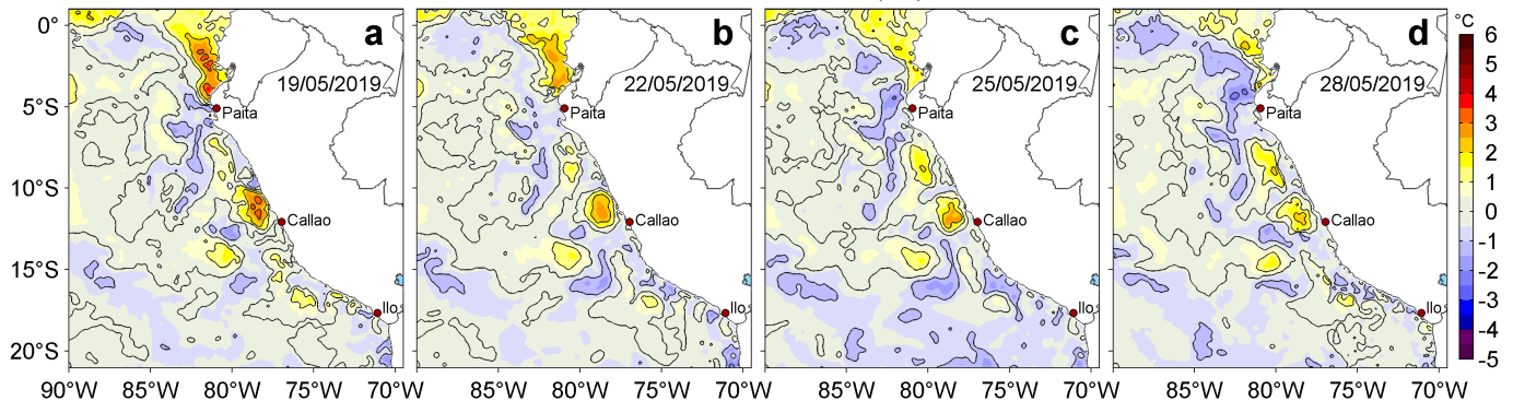
Figura 3. Anomalías de la temperatura superficial del mar (TSM, °C) para los días: a) 19, b) 22, c) 25 y d) 28 de mayo de 2019. Las anomalías se calcularon respecto de la climatología para el periodo 2007-2016. Datos: OSTIA-UKMO-L4-GLOB-v2.0 (UK Met Office, 2012; Donlon et al, 2012). Procesamiento: LHFM/AFIOF/DGIOCC/IMARPE.
