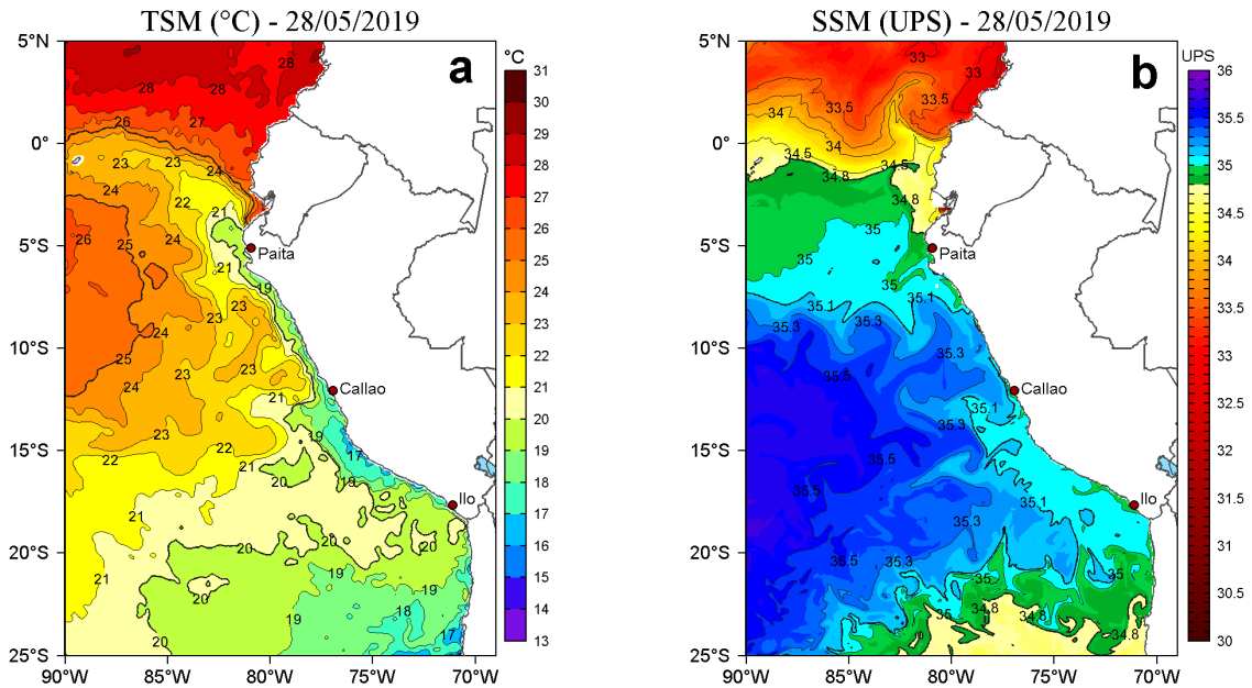
Figura 2. a) Temperatura superficial del mar (TSM, °C) y b) Salinidad superficial del mar (SSM, UPS), para el 28 de mayo de 2019. Datos: OSTIA-UKMO-L4-GLOB-v2.0 (UK Met Office, 2012; Donlon et al, 2012) disponible en https://podaac.jpl.nasa.gov/dataset/OSTIA-UKMO-L4-GLOB-v2.0 para (a) y Hybrid Coordinate Ocean Model v. GOF5 3.1 (HYCOM; Halliwell et al., 1998; 2000; Bleck, 2001) para (b). Procesamiento: LHFM/AFIOF/DGIOCC/IMARPE.
