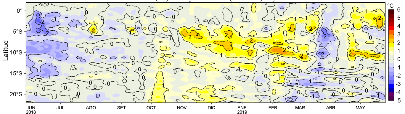
Figura 4. Variación promedio de las anomalías de la temperatura superficial del mar (TSM, °C) para una franja de 60 mn (~111 km) adyacente al litoral peruano para los últimos doce meses al 26 de mayo de 2019. Datos: OSTIA-UKMO-L4-GLOB-v2.0 (UK Met. Office, 2012; Donlon et al, 2012) disponible en https://podaac.jpl.nasa.gov/dataset/OSTIA-UKMO-L4-GLOB-v2.0 . Las anomalías se calcularon con respecto al periodo 2007-2016. Procesamiento: LHFM/AFIOF/DGIOCC/IMARPE.
