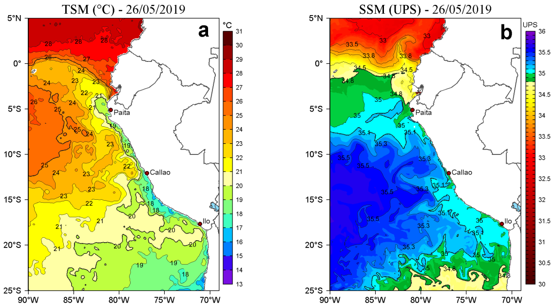
Figura 2. a) Temperatura superficial del mar (TSM, °C) y b) Salinidad superficial del mar (SSM, UPS), para el 26 de mayo de 2019. Datos: OSTIA-UKMO-L4-GLOB-v2.0 (UK Met Office, 2012; Donlon et al, 2012) disponible en https://podaac.jpl.nasa.gov/dataset/OSTIA-UKMO-L4-GLOB-v2.0 para (a) y Hybrid Coordinate Ocean Model v. GOF3 3.1 (HYCOM; Halliwell et al., 1998; 2000; Bleck, 2001) para (b). Procesamiento: LHFM/AFIOF/DGIOCC/IMARPE.
