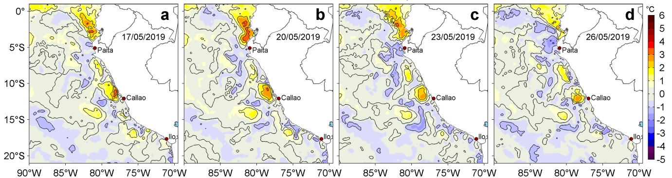
Figura 3. Anomalías de la temperatura superficial del mar (TSM, °C) para los días: a) 17, b) 20, c) 23 y d) 26 de mayo de 2019. Las anomalías se calcularon respecto de la climatología para el periodo 2007-2016. Datos: OSTIA-UKMO-L4-GLOB-v2.0 (UK Met Office, 2012; Donlon et al, 2012). Procesamiento: LHFM/AFIOF/DGIOCC/IMARPE.
